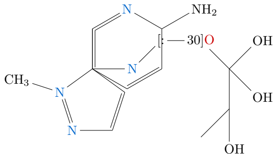
MESG
