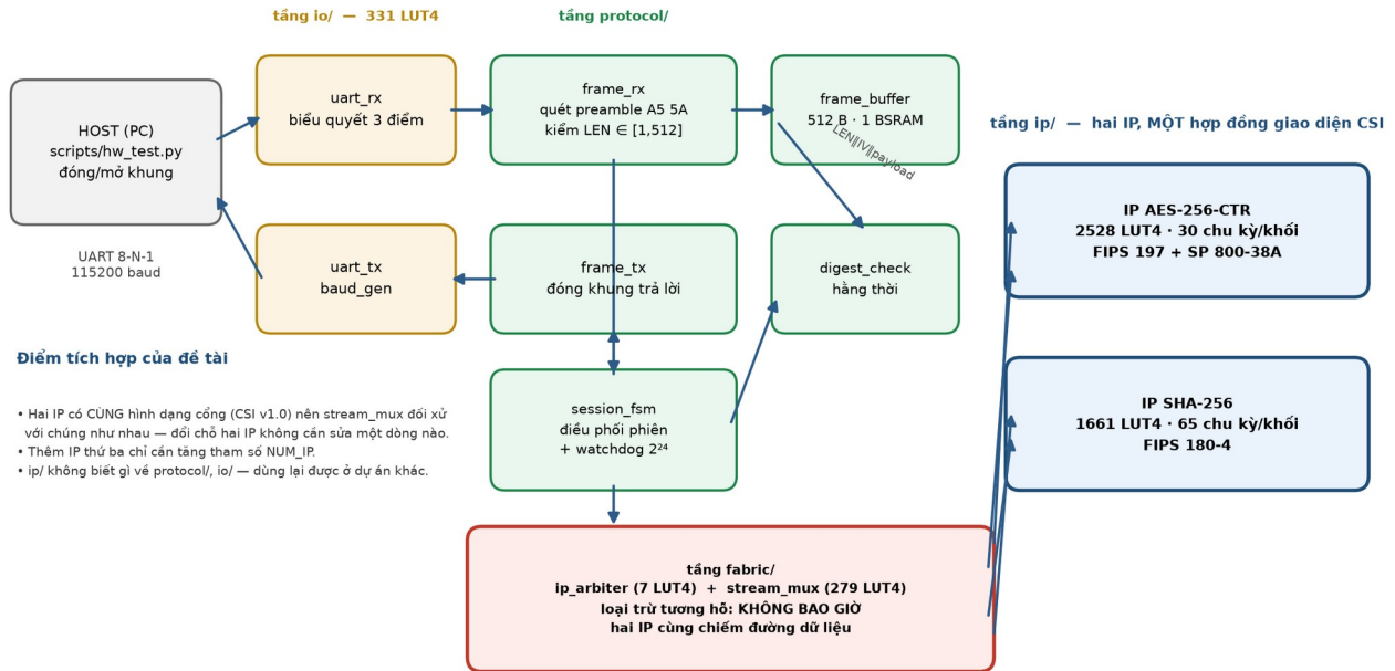
Hình 1. Kiến trúc bốn tầng, luồng dữ liệu một khung và số liệu tài nguyên đo được.
