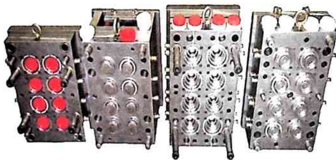
图13 不同尺寸的水瓶盖模具
