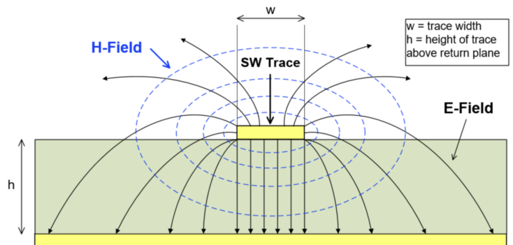
Abbildung 4.3.: Elektrisches und magnetisches Feld eines Leiterbahnschnitts [32]
