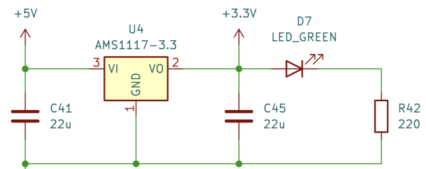
Abbildung 10.7.: Schaltplan des LDOs basierend auf dem AMS1117-3.3
