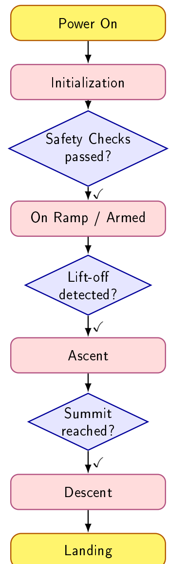
Abbildung 12.1.: Ablaufdiagramm des Raketenstarts
