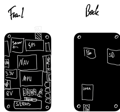
Abbildung 10.8.: Erste Skizze der Leiterplatte
