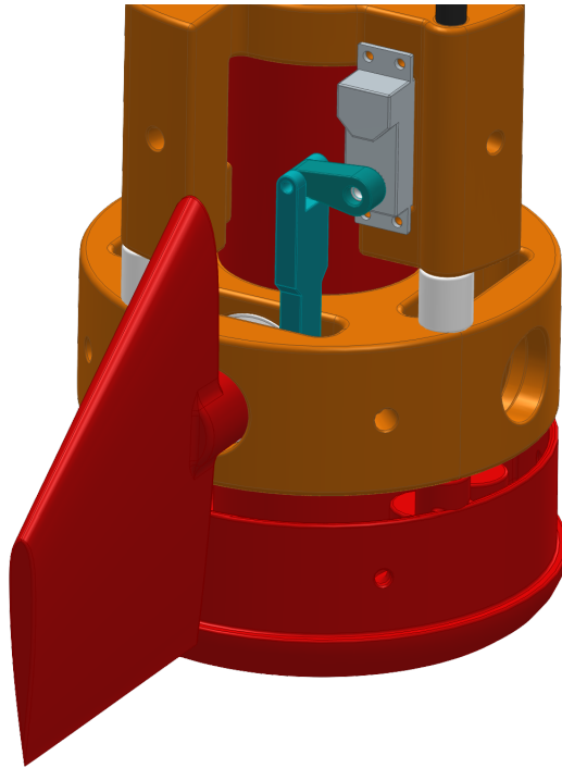
Abbildung 13.4.: Assembly des kompletten Finnensteuermechanismus
