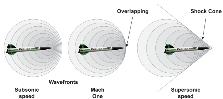
Abbildung 7.3.: Machscher Kegel [34]
