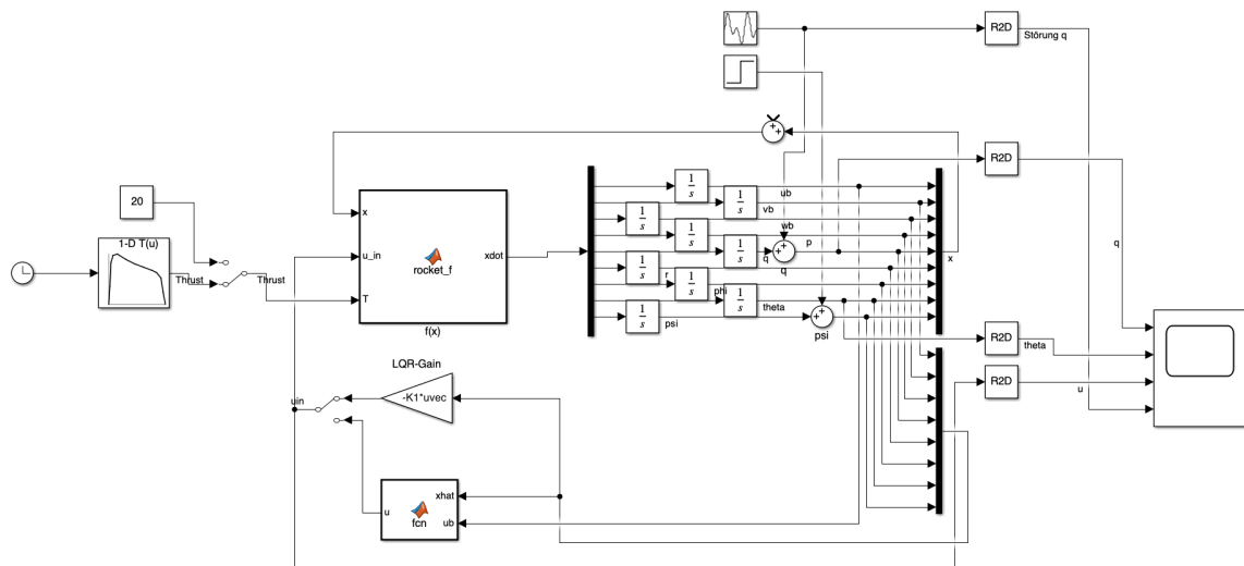
Abbildung D.1.: Simulink Modell der Rakete mit LQR-Regler für Abbildung 16.6
