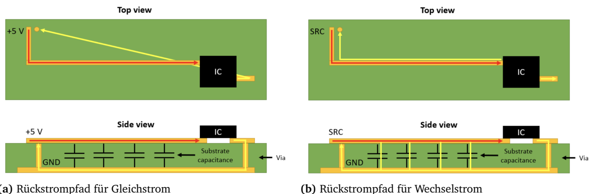
Abbildung 4.2.: Rückstrompfade im Vergleich [37]
