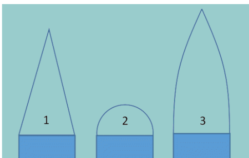
Abbildung 7.4.: Verschiedene Formen der Raketenspitze für Modellraketen bei Unterschallflug [26]
