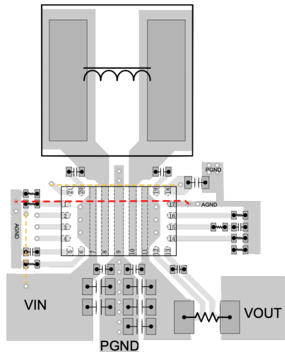
Abbildung 4.7.: Beispielhaftes Layout eines Abwärtswandlers [31]
