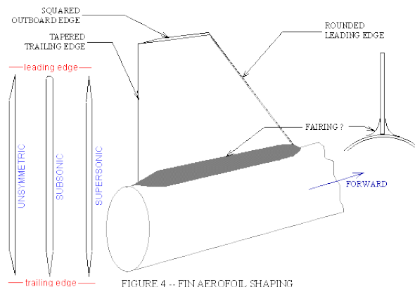
Abbildung 7.6.: Flügelprofile [NakkaRocketry]
