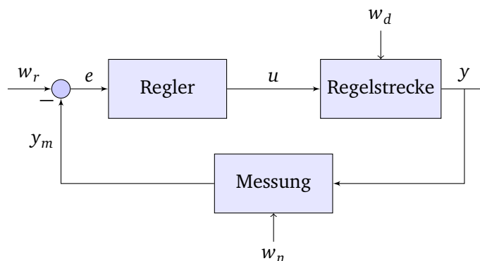
Abbildung 6.2.: Standard-Regelkreis
