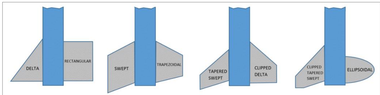
Abbildung 7.3.: Verschiedene Flügelformen [15]
