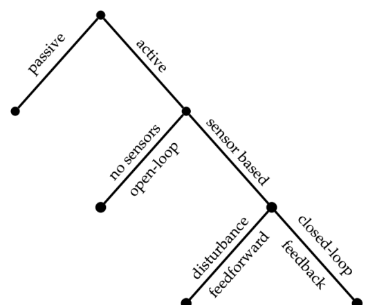
Abbildung 6.1.: Arten von Systemsteuerung [16]
