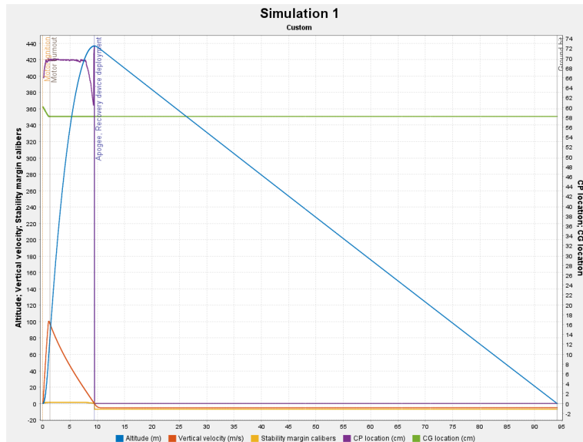
Abbildung 15.1.: Plot von den aus OpenRocket bezogenen Werten
