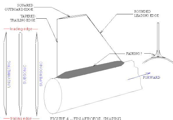
Abbildung 7.4.: Flügelprofile [16]
