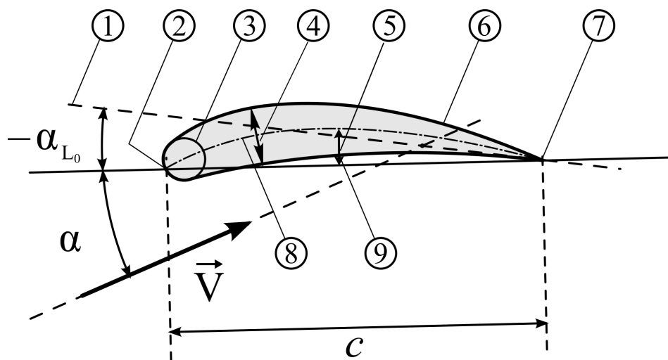
Abbildung 7.5.: Geometrie der NACA Profile [21]
