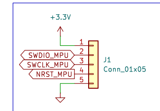
DEBUG_NAV
