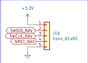
DEBUG_NAV
