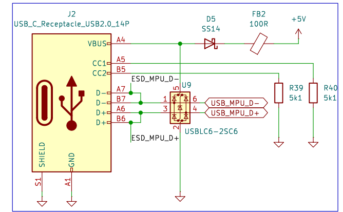
USB MPU
