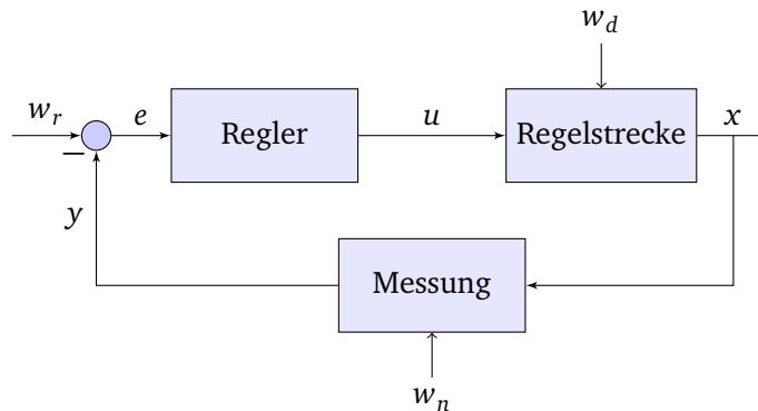
Abbildung 6.1.: Standard-Regelkreis
