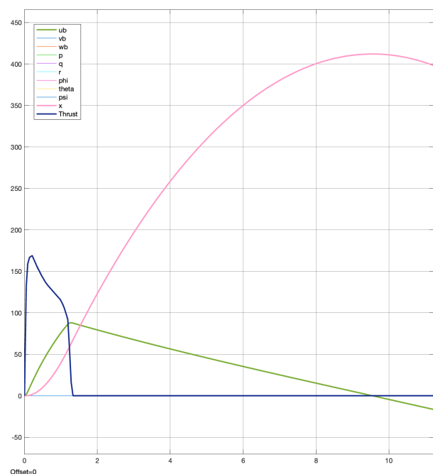
Abbildung 16.1.: Ungestörter Flug der Rakete mit einem H-Motor
