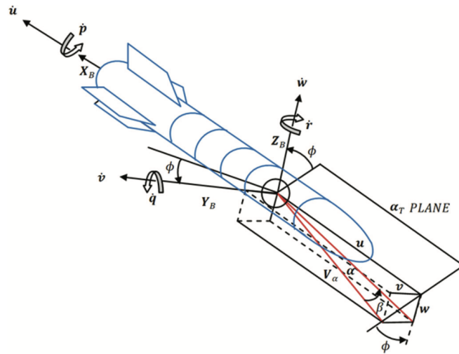
Abbildung 9.1.: Modell einer Rakete mit 6 Freiheitsgraden [8]
