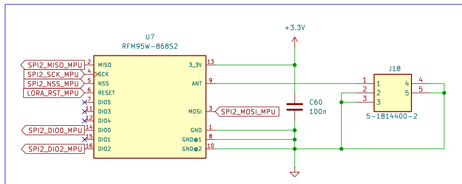
LORA Module
