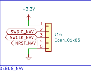
DEBUG_NAV
