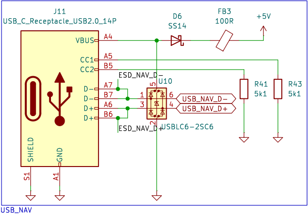
USB_NAV
