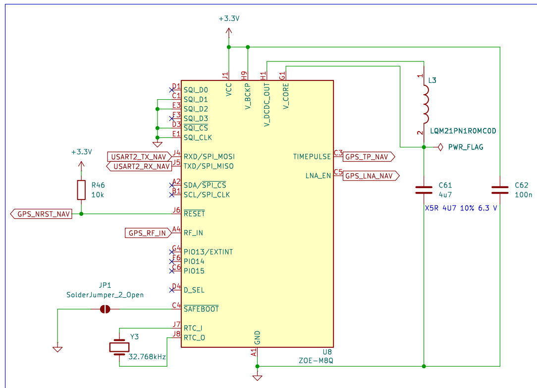
GNSS Modul
