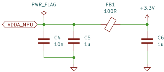
Abbildung 9.3.: PI-Filter zur Entkopplung der VDDA und VREF+ Pins von der 3.3V Schiene
