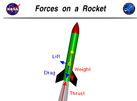
Abbildung 7.1.: Die 4 wichtigsten Kräfte auf einen Raketenflugkörper [14]
