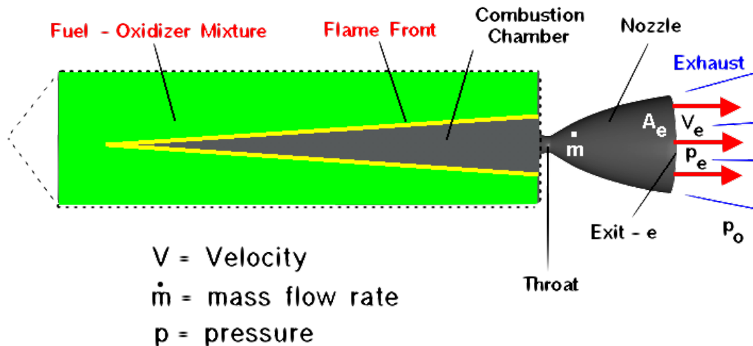
Abbildung 8.2.: Aufbau eines Feststofftriebwerks [15]
