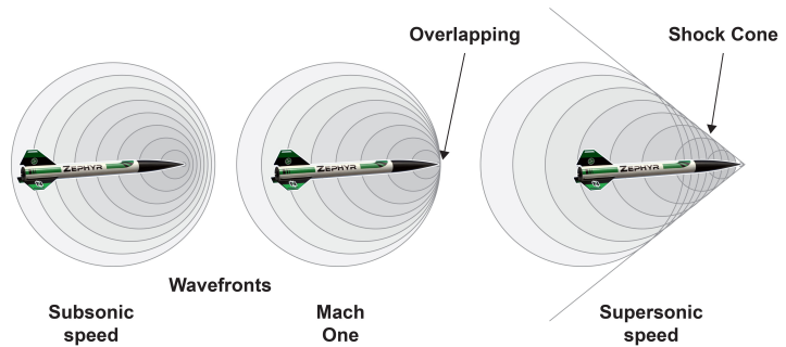
Abbildung 7.3.: Machscher Kegel [35]
