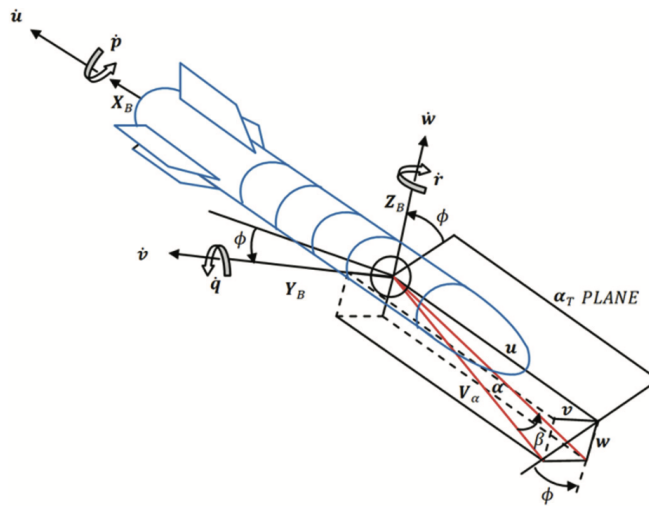
Abbildung 10.2.: Modell einer Rakete mit 6 Freiheitsgraden [12]
