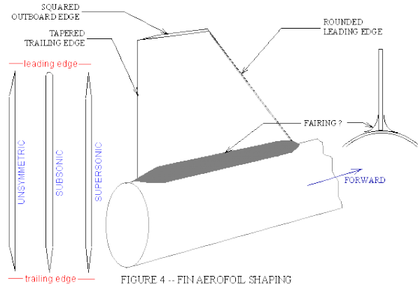
Abbildung 7.4.: Flügelprofile [15]
