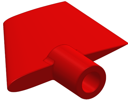
Abbildung 14.8.: CAD-Modell des Raketenflügels zur Befestigung im Windkanal
