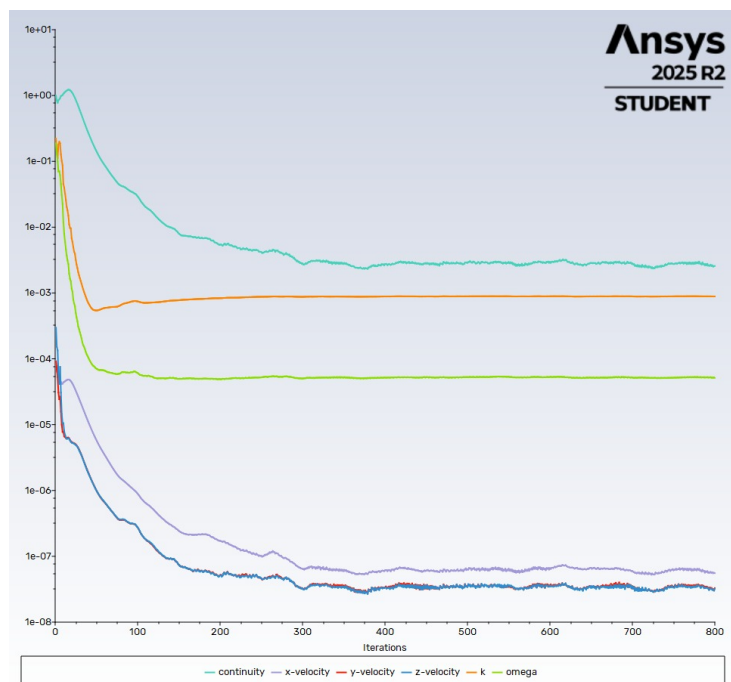
Abbildung 14.2.: Plot der Residuals im 8. Simulationsfall
