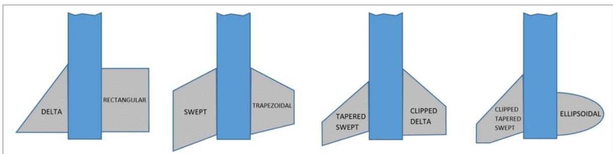
Abbildung 7.5.: Verschiedene Flügelformen [27]
