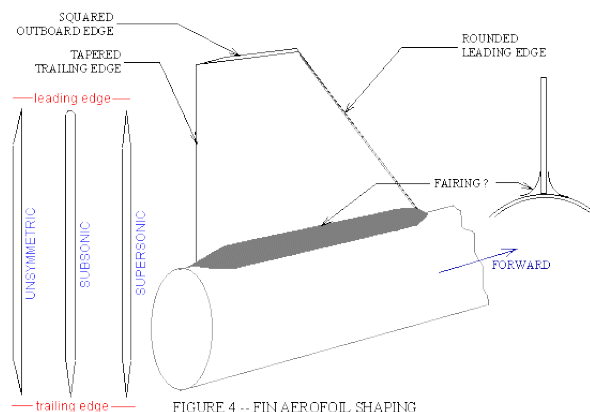
Abbildung 7.6.: Flügelprofile [27]
