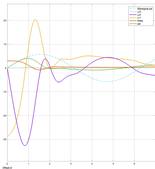
Abbildung 16.5.: Verlauf mit Nachführung der K -Matrix
