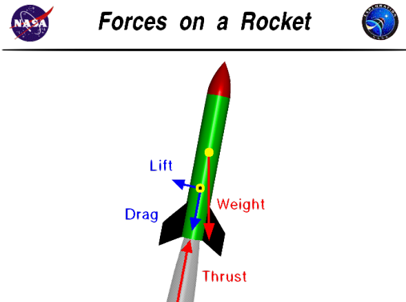
Abbildung 7.1.: Die 4 wichtigsten Kräfte auf einen Raketenflugkörper [14]
