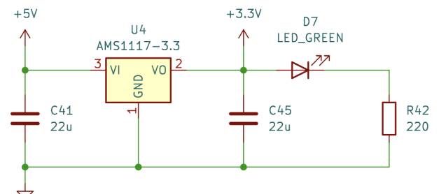
Abbildung 10.7.: Schaltplan des LDOs basierend auf dem AMS1117-3.3
