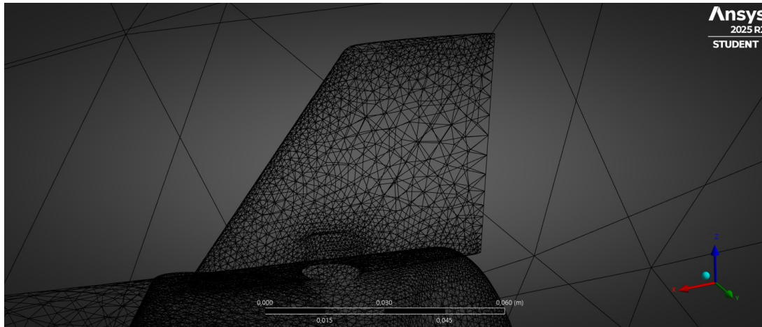
Abbildung 14.1.: Vernetzter Raketenflügel
