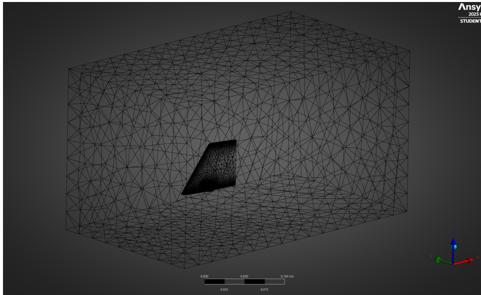
Abbildung 8.1.: Mesh der Geometrie in Ansys Mechanical
