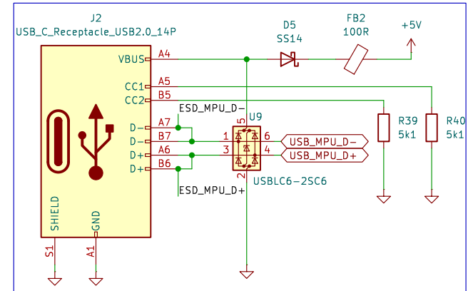
USB_MPU
