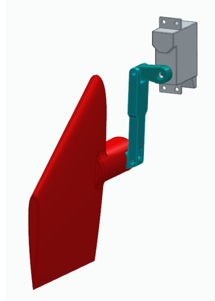
Abbildung 12.2.: Flügelsteuermechanismus
