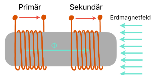
Abbildung 4.10.: Funktionsprinzip eines Fluxgate-Magnetometers
