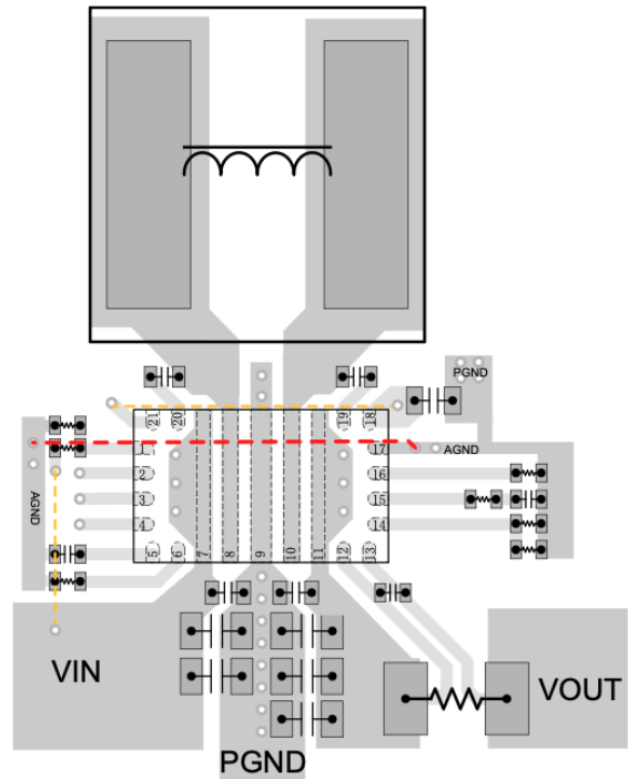
Abbildung 4.6.: Beispielhaftes Layout eines Abwärtswandlers [10]
