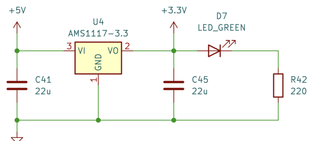
Abbildung 9.7.: Schaltplan des LDOs basierend auf dem AMS1117-3.3
