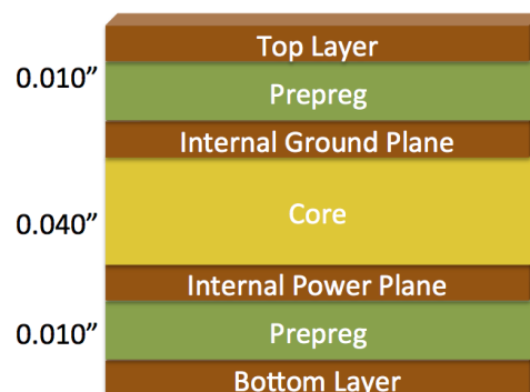
Abbildung 4.1.: Beispielhafter Stackup einer vierlagigen Leiterplatte [14]
