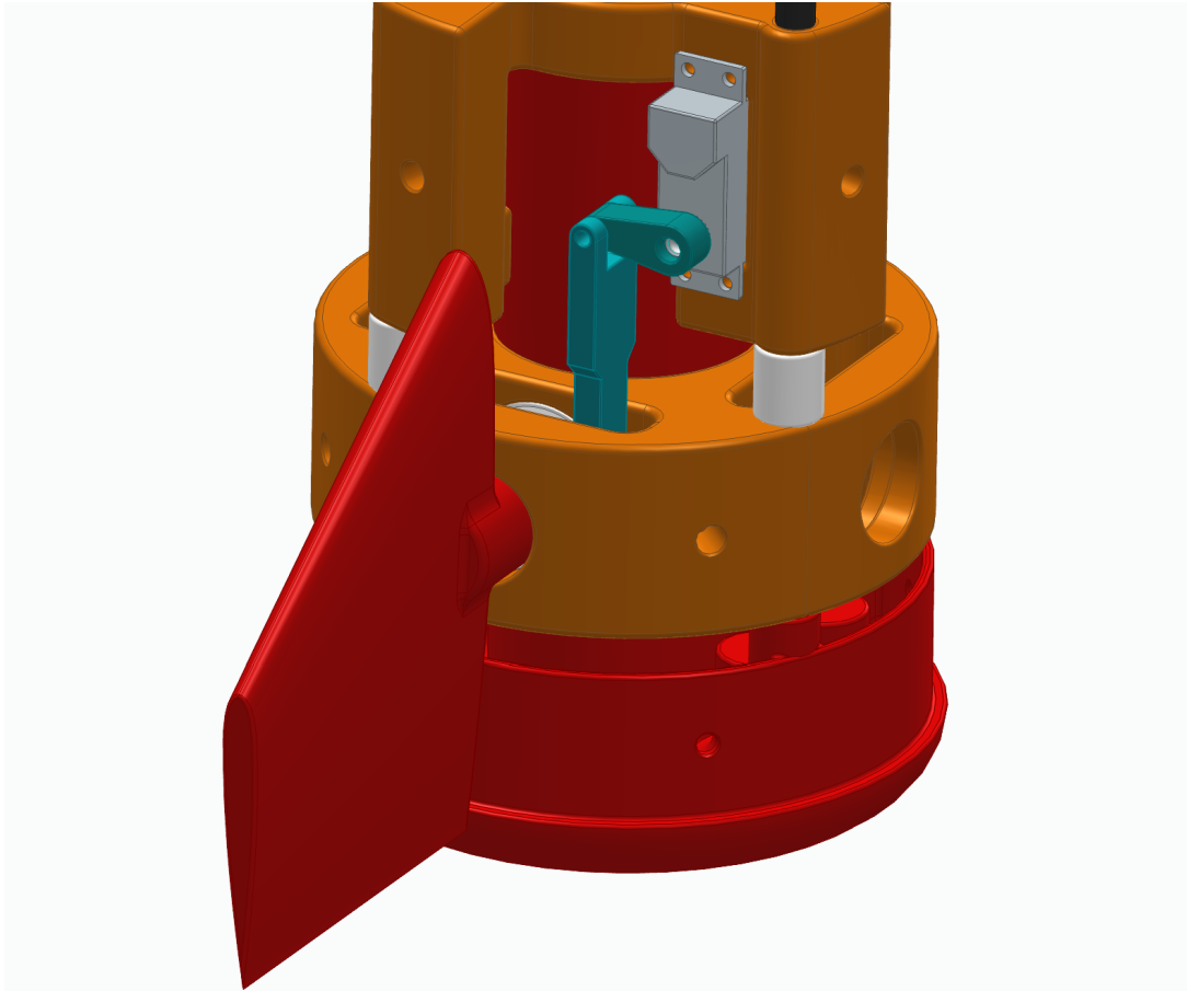
Abbildung 12.4.: Assembly des kompletten Finnensteuermechanismus
