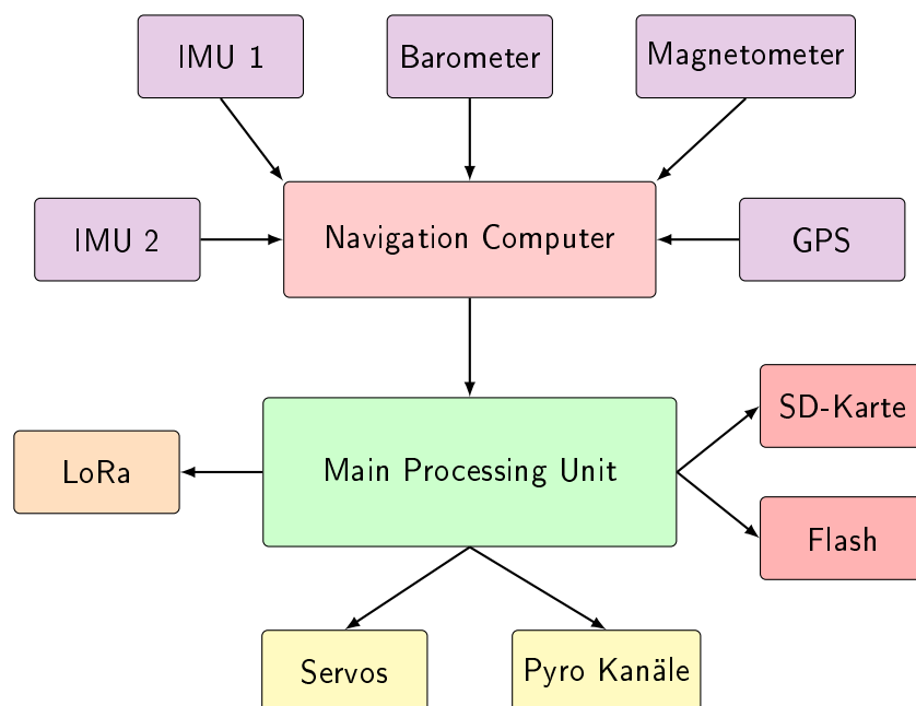
Abbildung 9.1.: Systemarchitektur des Flightcomputers
