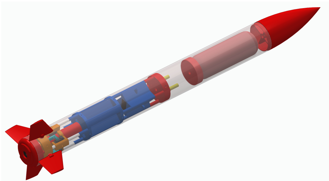
Abbildung 12.7.: Solid Edge Assembly
