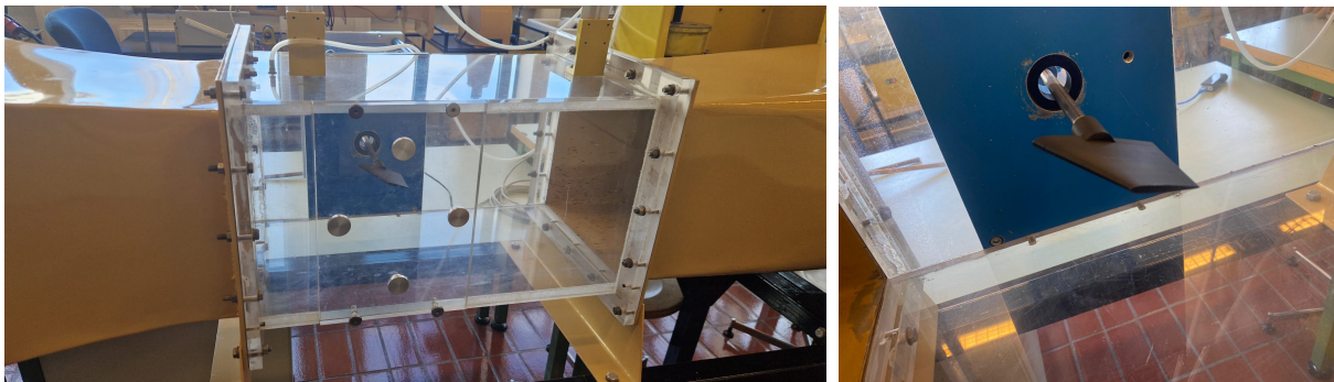
Abbildung 13.9.: Messaufbau vom Raketenflügel im Windkanal
