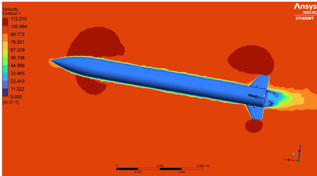
Abbildung 13.5.: Geschwindigkeit am Raketenkörper
