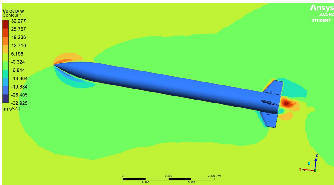
Abbildung 13.6.: Z-Komponente der Geschwindigkeit am Raketenkörper
