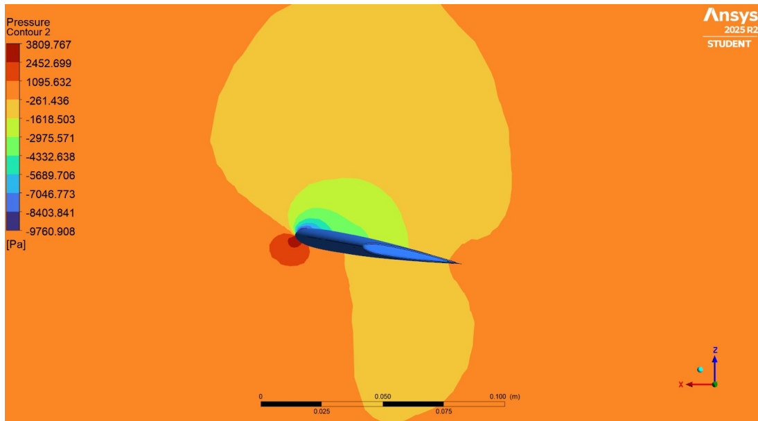
Abbildung 13.2.: Druck am Raketenflügel
