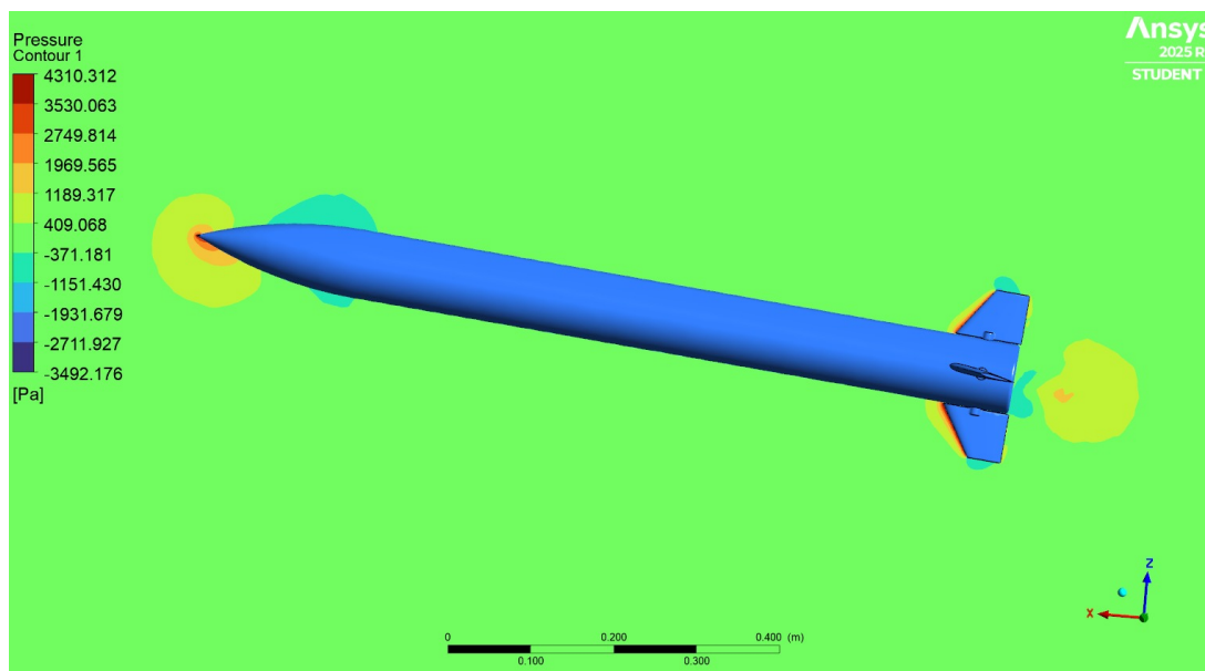
Abbildung 13.4.: Druck am Raketenkörper
