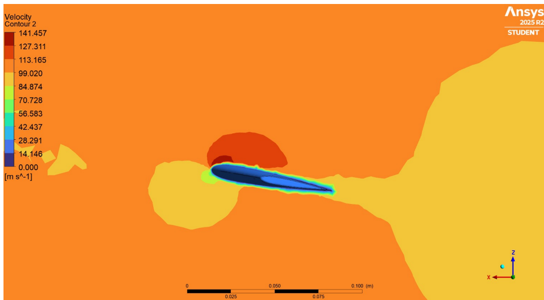
Abbildung 13.3.: Geschwindigkeit am Raketenflügel
