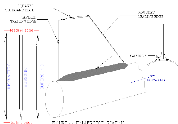
Abbildung 7.4.: Flügelprofile [16]
