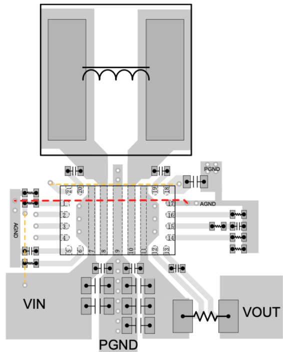
Abbildung 4.7.: Beispielhaftes Layout eines Abwärtswandlers [15]
