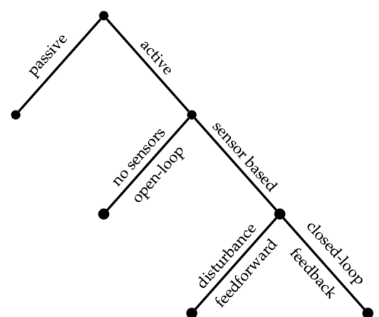
Abbildung 6.1.: Arten von Systemsteuerung [14]
