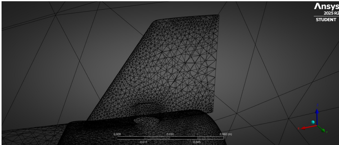
Abbildung 13.1.: Vernetzter Raketenflügel
