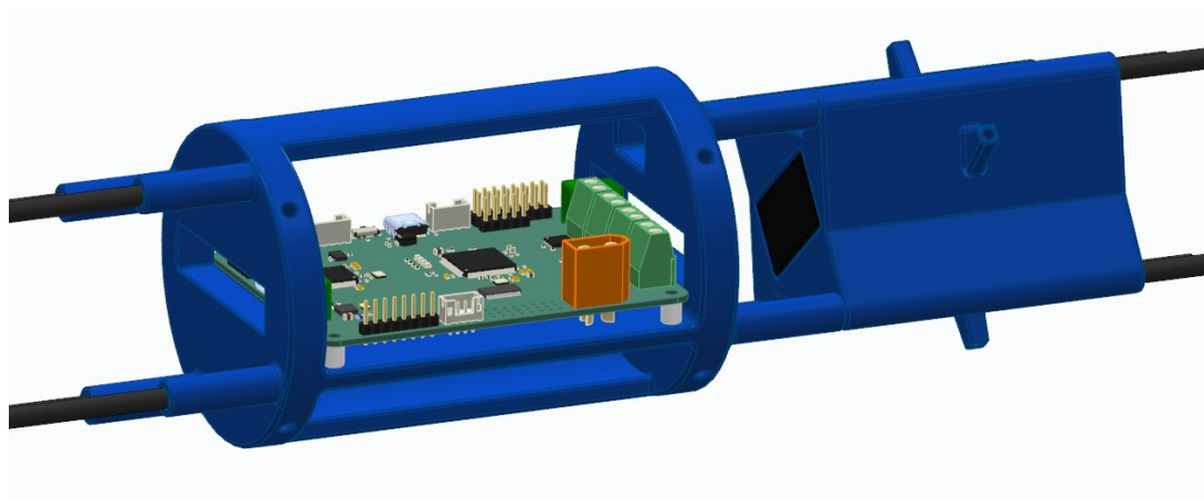
Abbildung 12.4.: Montierung vom Flightcomputer und Akku
