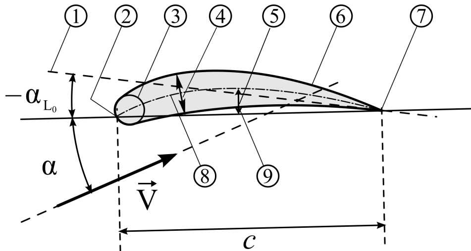
Abbildung 7.4.: Geometrie der NACA Profile [21]
