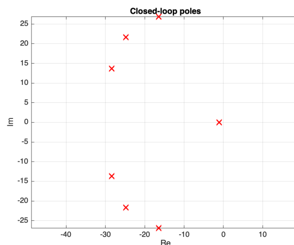
Abbildung 6.3: Eigenwerte eines stabilen geschlossenen Regelkreises
