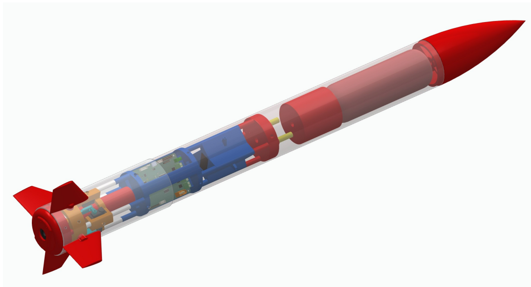
Abbildung 12.8: Zusammengesetzte CAD-Baugruppe der Rakete
