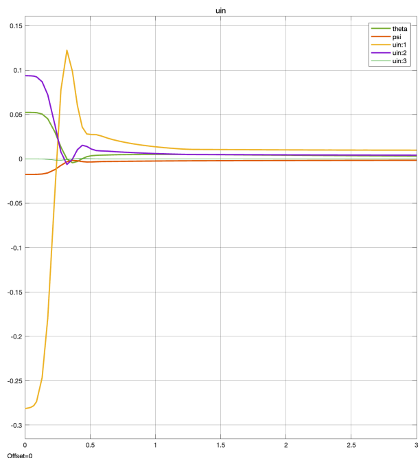
Abbildung 15.3: Ungestörter Flug der Rakete mit einem H-Motor
