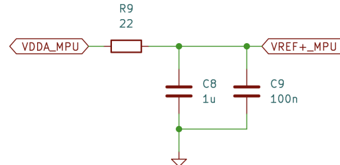
Abbildung 9.4: RC-Tiefpass zur Stabilisierung der Referenzspannung am VREF+ Pin
