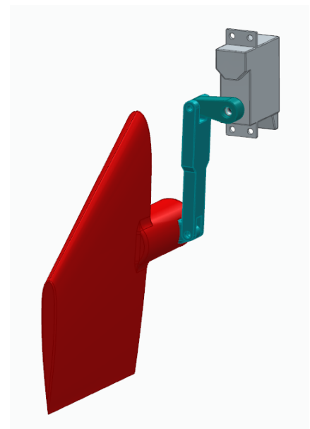
Abbildung 12.2: Gelenksystem zur Flügelsteuerung
