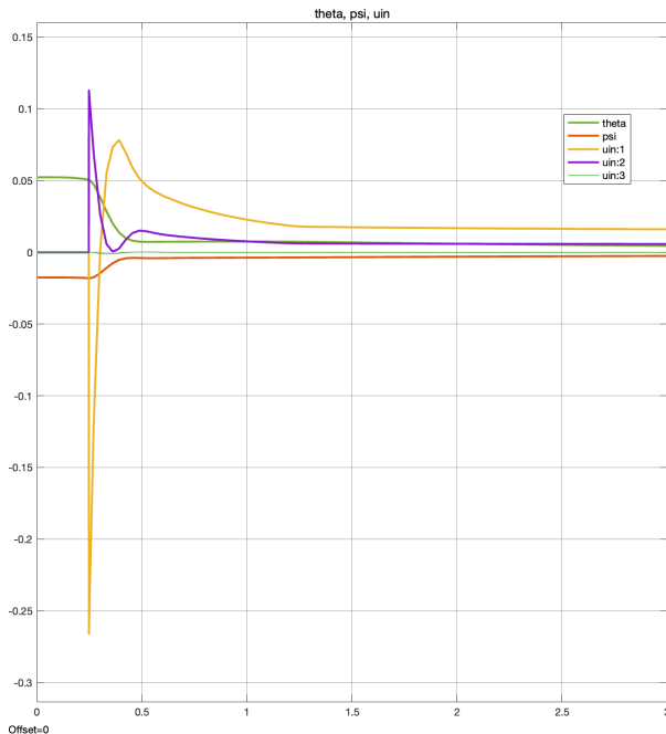
Abbildung 15.2: Ungestörter Flug der Rakete mit einem H-Motor. Im Vergleich dazu ist in Abbildung ?? die Simulation des gleichen Fluges dargestellt, bei dem die Regelung von Anfang an aktiv ist und die K-Matrix für die Geschwindigkeit von 50 \frac{m}{s} verwendet wird. Es ist zu erkennen, dass sich die beiden Verläufe grundsätzlich sehr ähnlich sind, die Auslenkung der Finnen jedoch merklich größer ist was zu einem Überschwinger des Winkels \theta führt. In diesem Fall ist das in Ordnung und führt zu keinerlei Problemen, da die Regelung ohnehin im Bereich unter 50 \frac{m}{s} bis ca. 1 s bleibt siehe Abbildung ??.
