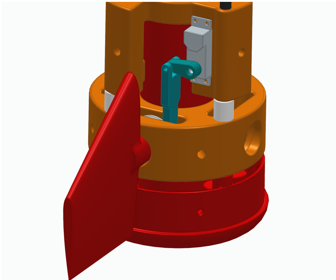
Abbildung 12.4: Assembly des kompletten Finnensteuermechanismus
