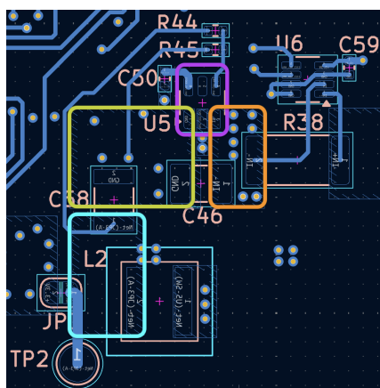
Abbildung 9.11: Vergleich des Layouts des Buck Converters mit einem Referenzlayout des Herstellers
