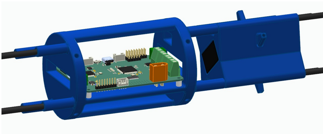
Abbildung 12.5: Montierung vom Flightcomputer und Akku
