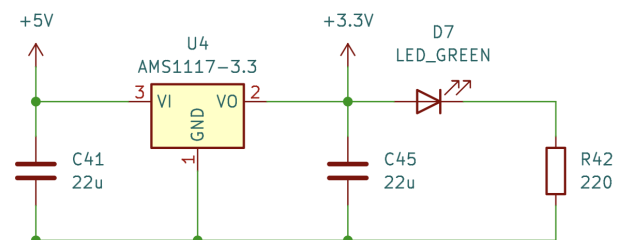
Abbildung 9.7.: Schaltplan des LDOs basierend auf dem AMS1117-3.3
