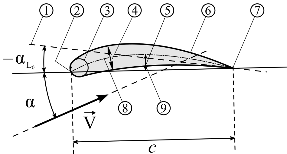
Abbildung 7.6.: Geometrie der NACA Profile [31]
