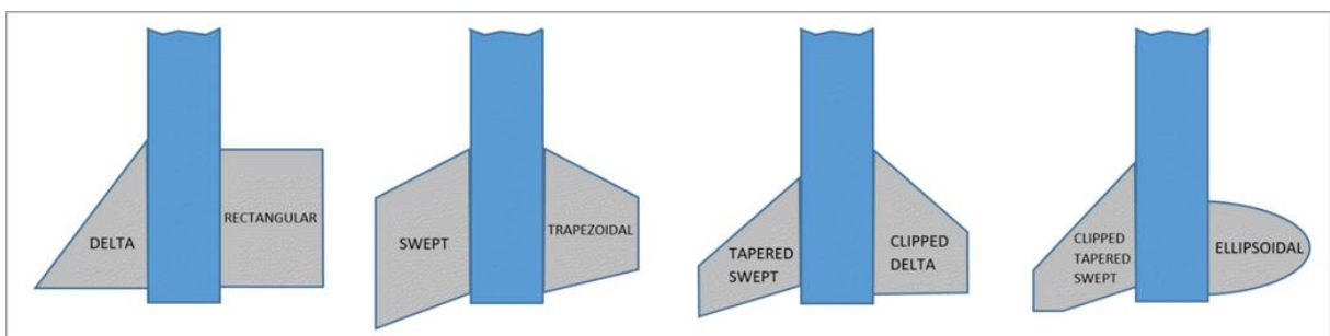
Abbildung 7.4.: Verschiedene Flügelformen [21]
