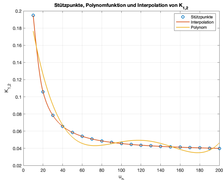
Abbildung 10.3.: Vergleich der Polynomfunktion mit Interpolation des Eintrags k_{12} der K-Matrix
