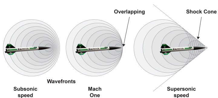
Abbildung 7.2: Machscher Kegel [19]
