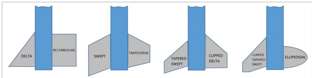
Abbildung 7.3: Verschiedene Flügelformen [15]
