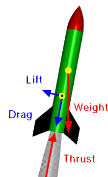
Abbildung 7.1.: Die 4 wichtigsten Kräfte auf einen Raketenflugkörper [14]
