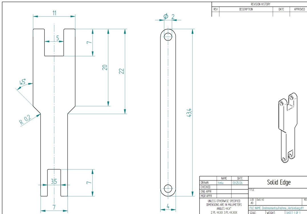
Abbildung 14.11.: Zeichnung der Gelenkverbindung beider Hebel des Flügelsteuermechanismus
