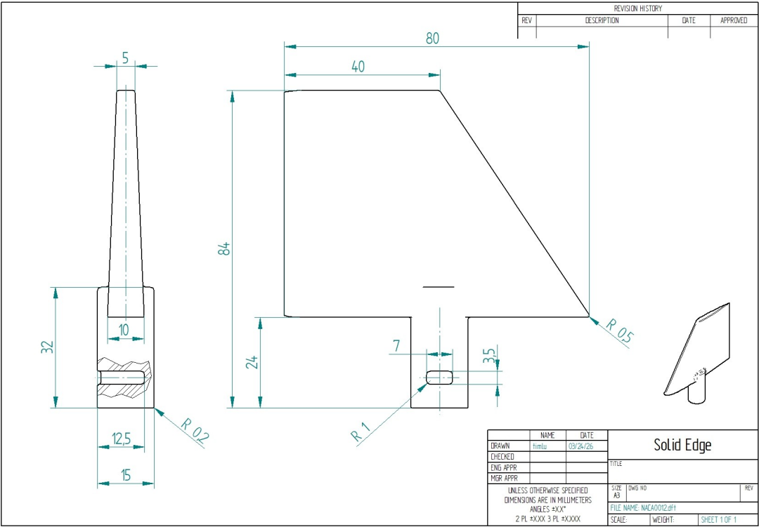
Abbildung 14.2.: Zeichnung des Raketenflügels
