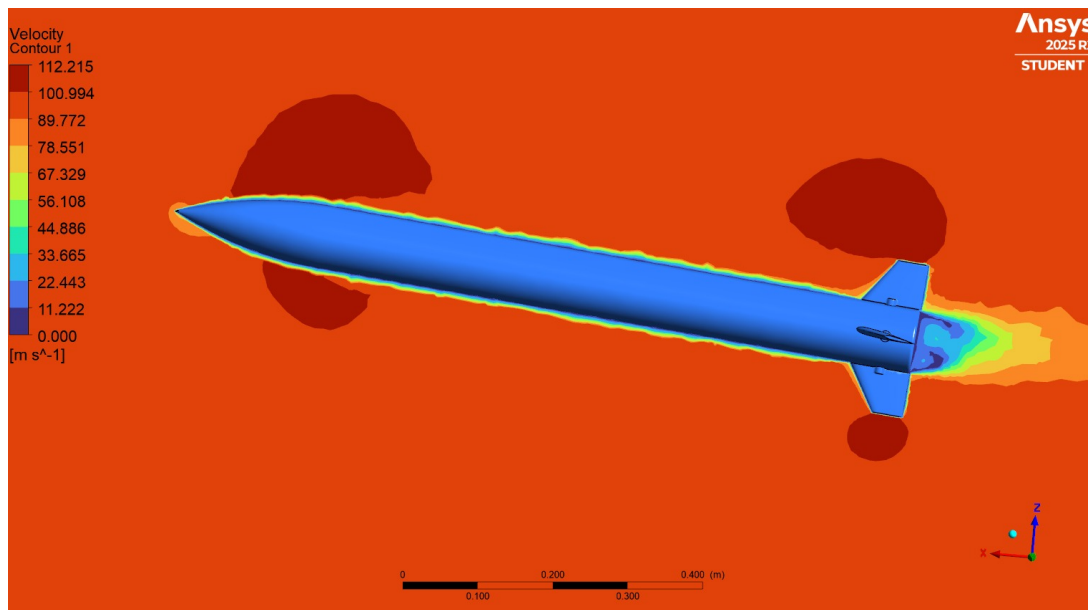
Abbildung 13.6.: Geschwindigkeit am Raketenkörper
