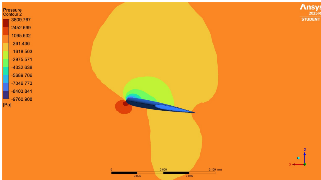
Abbildung 13.3.: Druck am Raketenflügel
