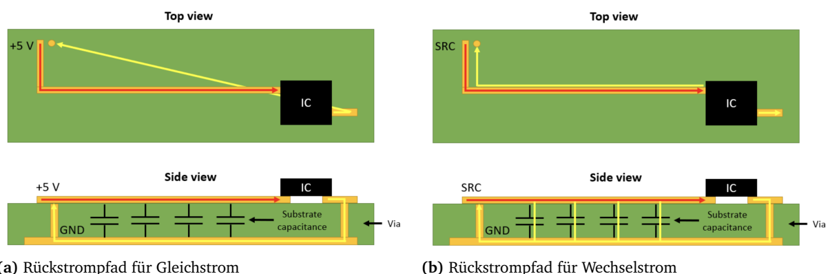
Abbildung 4.2.: Rückstrompfade im Vergleich [33]
