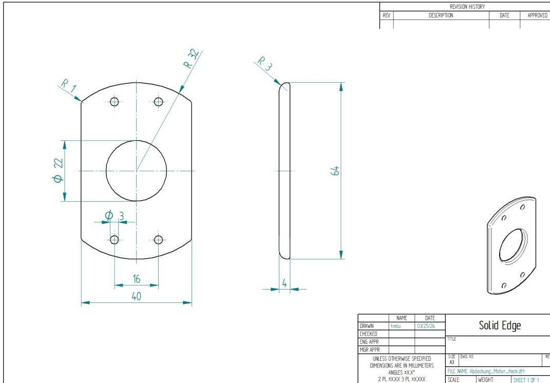
Abbildung 14.7.: Zeichnung der Motorabdeckung an der Motorhalterung
