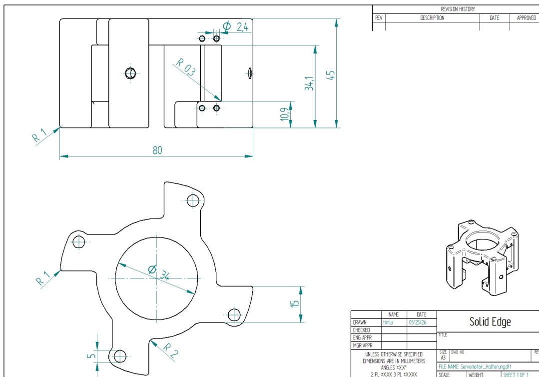
Abbildung 14.8.: Zeichnung der Servomotorhalterung
