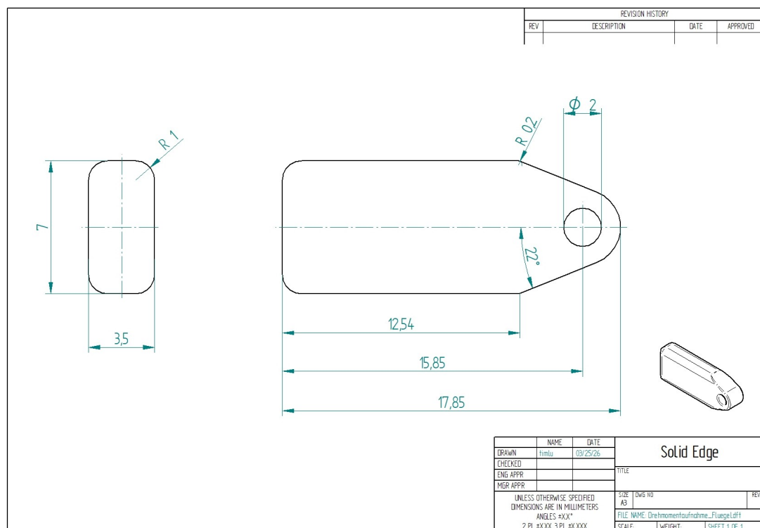
Abbildung 14.10.: Zeichnung des Flügelsteuermechanismushebels am Flügel
