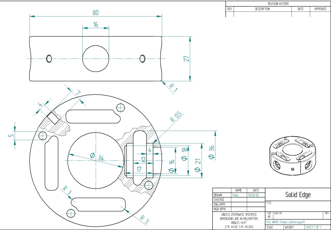
Abbildung 14.6.: Zeichnung der Flügelhalterung
