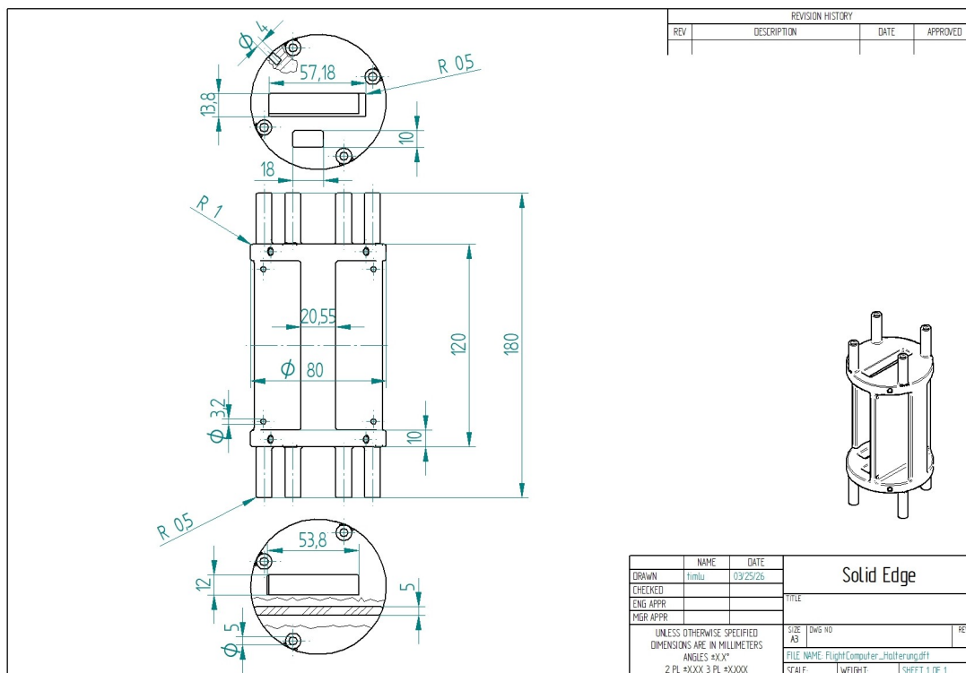
Abbildung 14.12.: Zeichnung der Halterung des Flightcomputers
