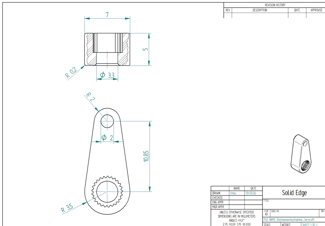
Abbildung 14.9.: Zeichnung des Flügelsteuermechanismushebels am Servomotor
