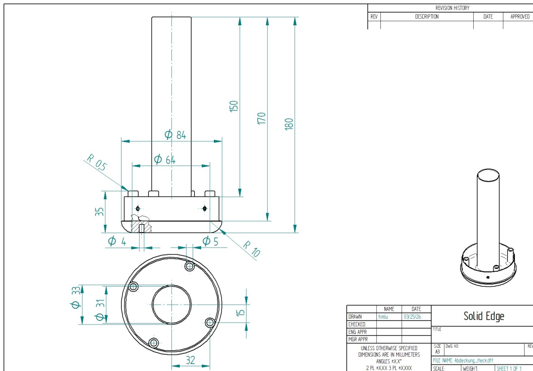
Abbildung 14.3.: Zeichnung der hinteren Abdeckung/Motorhalterung
