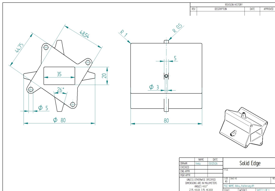
Abbildung 14.4.: Zeichnung der Akkuhalterung
