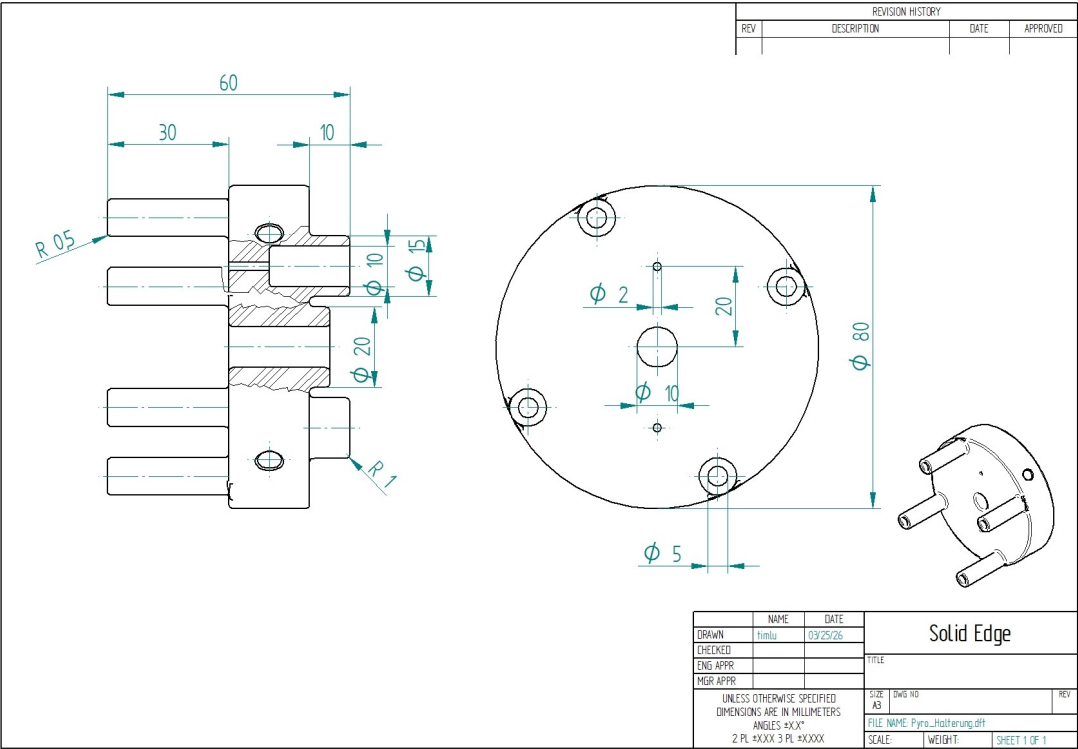
Abbildung 14.5.: Zeichnung der Halterung der Bergungssystemzündler
