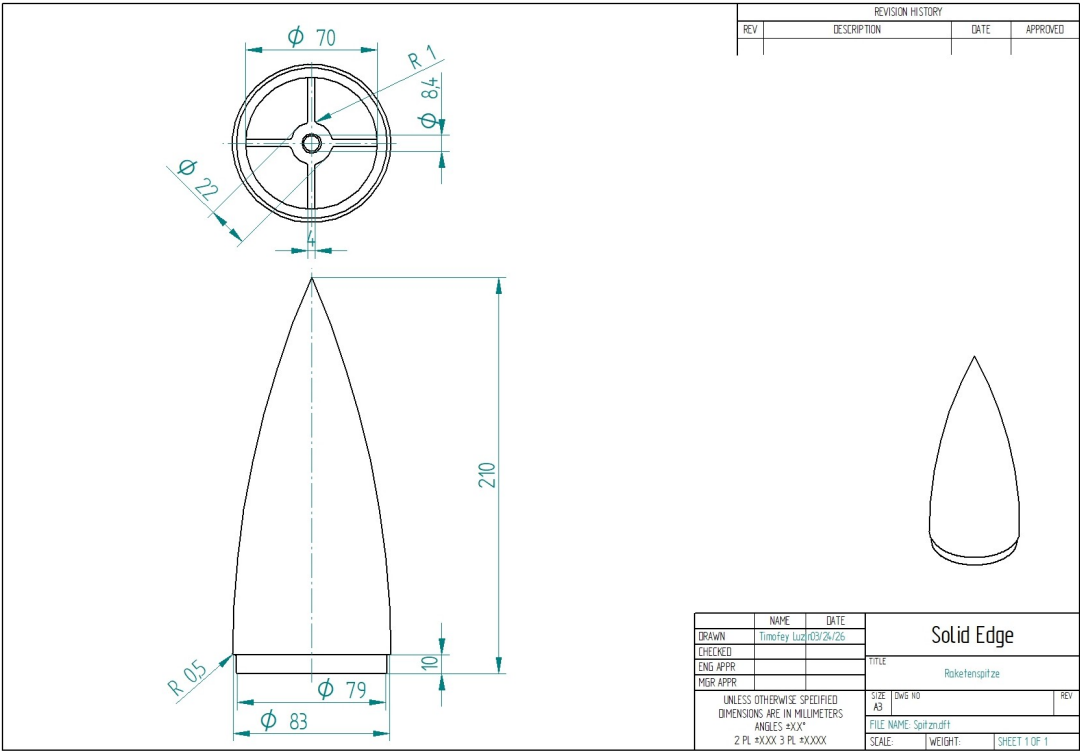
Abbildung 14.1.: Zeichnung der Raketenspitze
