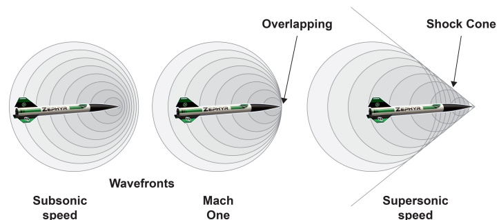
Abbildung 7.2.: Machscher Kegel [30]
