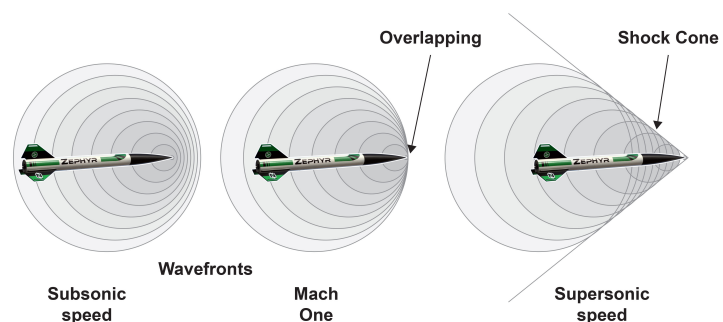
Abbildung 7.2.: Machscher Kegel [25]
