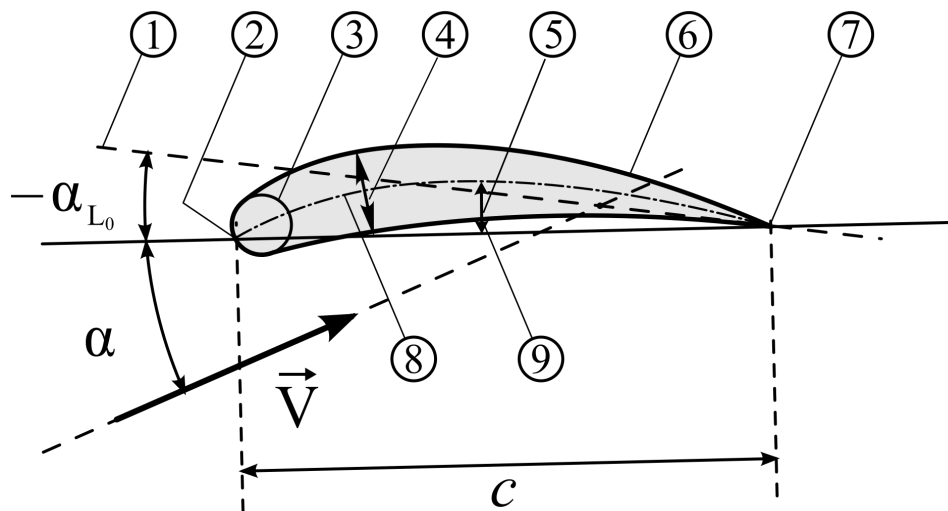
Abbildung 7.6.: Geometrie der NACA Profile [27]
