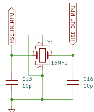
Abbildung 9.5.: Quarzschwingkreis zur Taktfrequenzgenerierung
