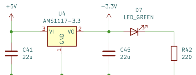
Abbildung 10.7.: Schaltplan des LDOs basierend auf dem AMS1117-3.3
