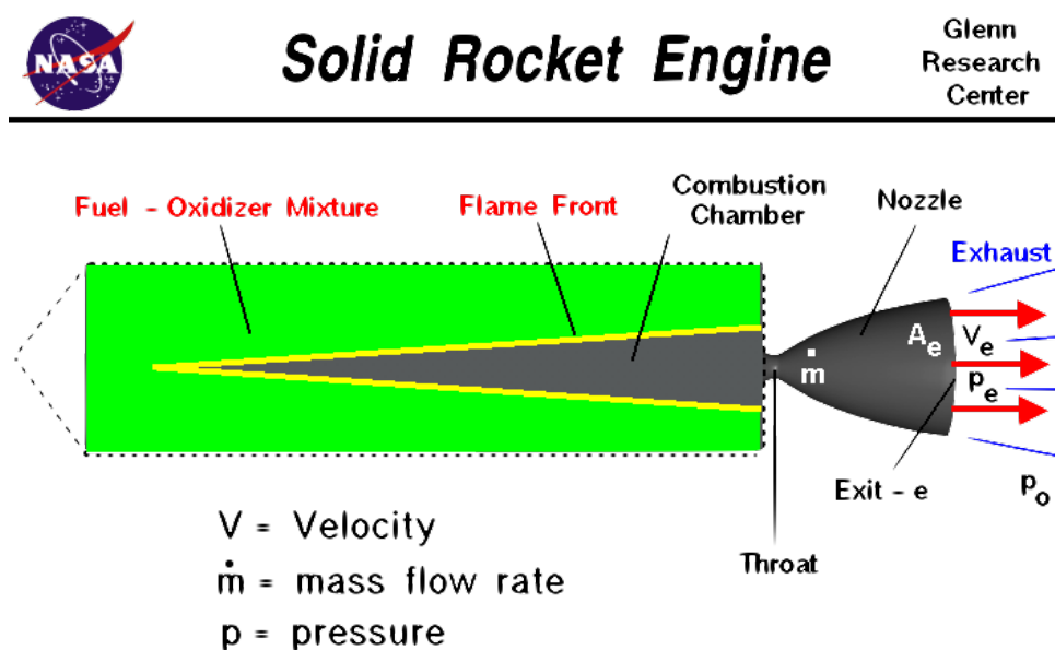
Abbildung 9.1.: Aufbau eines Feststofftriebwerks [13]
