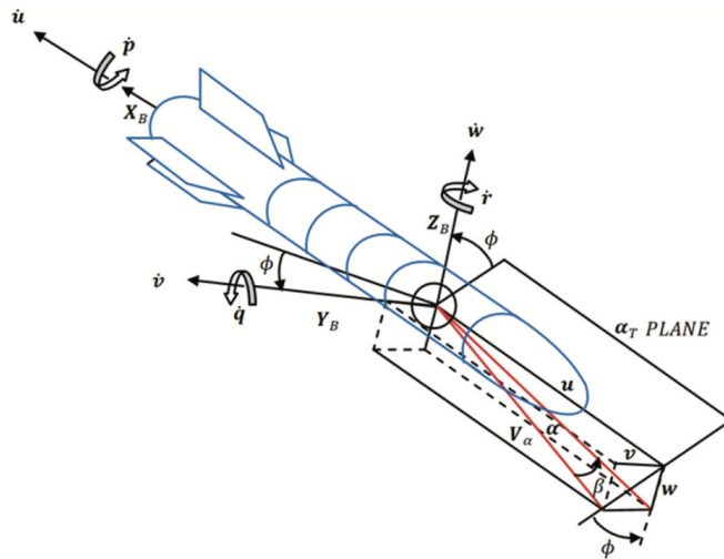
Abbildung 11.2.: Modell einer Rakete mit 6 Freiheitsgraden [10]
