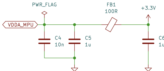
Abbildung 10.3.: PI-Filter zur Entkopplung der VDDA und VREF+ Pins von der 3.3 V Schiene
