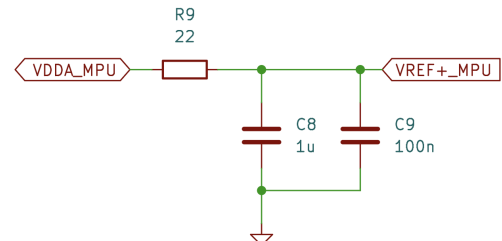
Abbildung 10.4.: RC-Tiefpass zur Stabilisierung der Referenzspannung am VREF+ Pin
