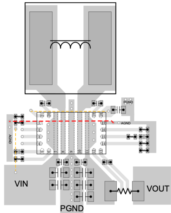
Abbildung 4.6.: Beispielhaftes Layout eines Abwärtswandlers [13]
