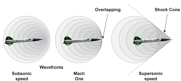
Abbildung 7.2.: Machscher Kegel [8]
