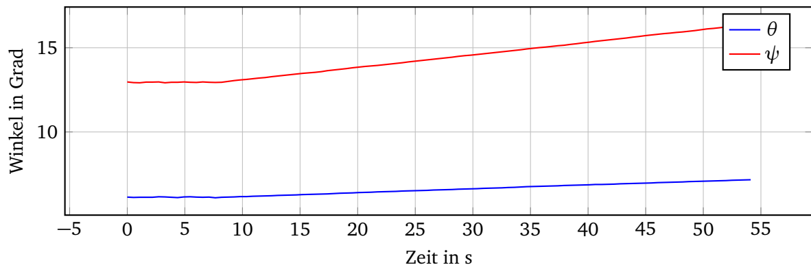
Abbildung 16.8: Verlauf der Winkel \theta und \psi ohne Updateschritt durch Beschleunigungsdaten
