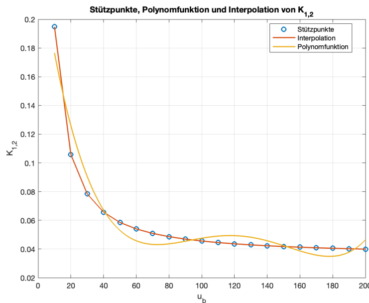
Abbildung 11.3: Vergleich der Polynomfunktion mit Interpolation des Eintrags k_{12} der \mathbf{K} -Matrix
