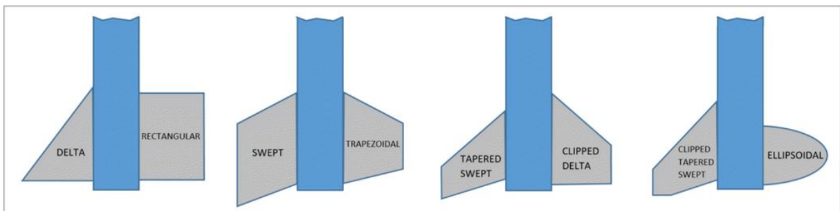
Abbildung 7.5: Verschiedene Flügelformen [26]
