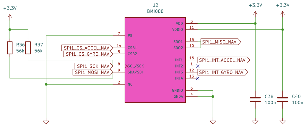
Abbildung 10.2: Schaltplan des BMI088
