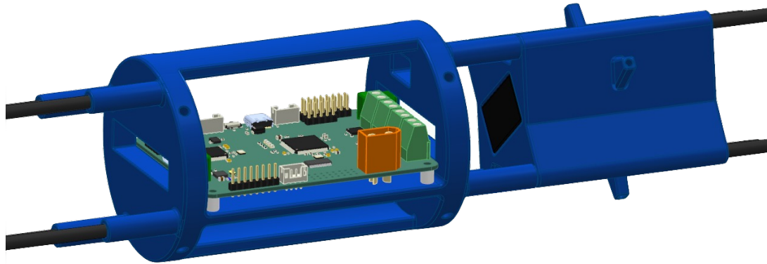
Abbildung 13.5: Montage des Flightcomputer und Akku
