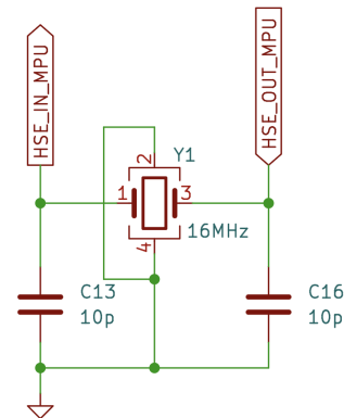
Abbildung 10.5: Quarzschwingkreis zur Taktfrequenzgenerierung
