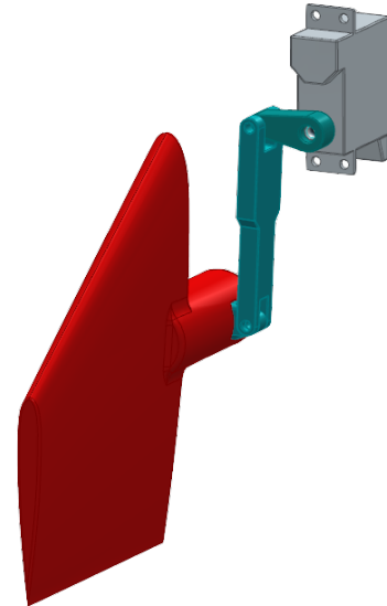
Abbildung 13.2: Gelenksystem zur Flügelsteuerung
