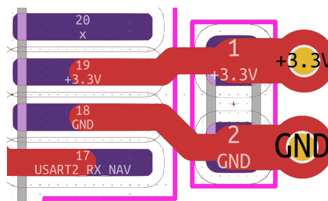
Abbildung 4.4: Platzierung von Decoupling-Kondensatoren
