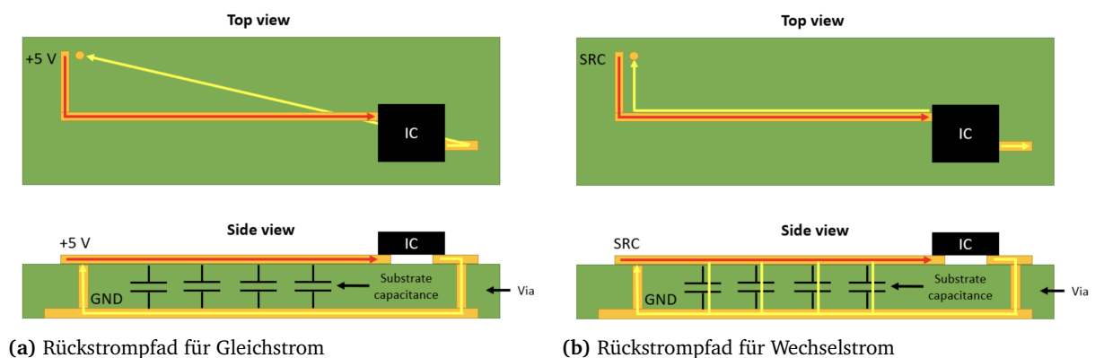
Abbildung 4.2: Rückstrompfade im Vergleich [38]
