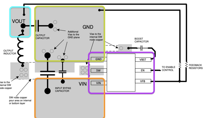
Abbildung 10.11: Vergleich des Layouts des Buck Converters mit einem Referenzlayout des Herstellers
