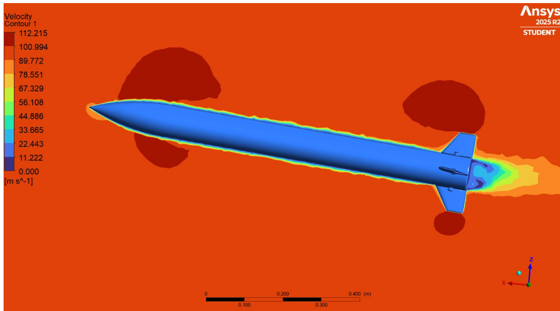
Abbildung 14.6: Geschwindigkeit am Raketenkörper
