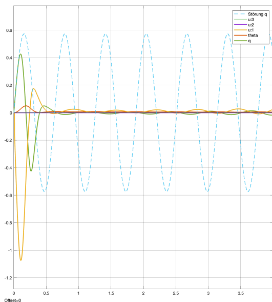
Abbildung 16.5: Verlauf mit Nachführung der K-Matrix
