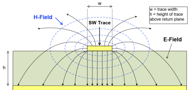
Abbildung 4.3: Elektrisches und magnetisches Feld eines Leiterbahnschnitts [33]
