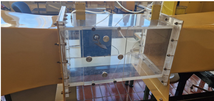
Abbildung 14.9: Messaufbau vom Raketenflügel im Windkanal
