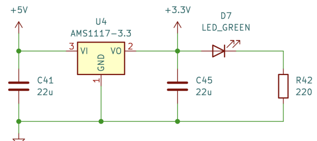
Abbildung 10.7: Schaltplan des LDOs basierend auf dem AMS1117-3.3
