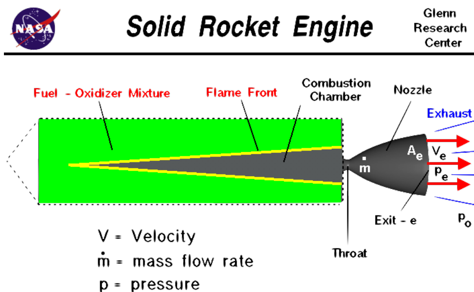
Abbildung 9.1: Aufbau eines Feststofftriebwerks [15]
