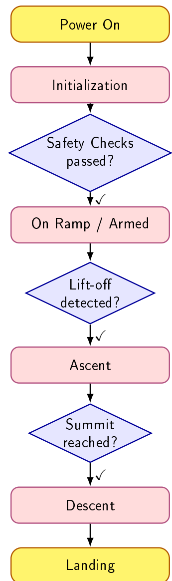
Abbildung 12.1: Ablaufdiagramm des Starts
