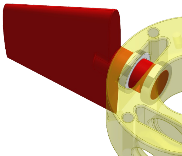
Abbildung 13.3: Befestigung des Raketenflügels mit Kugellagern
