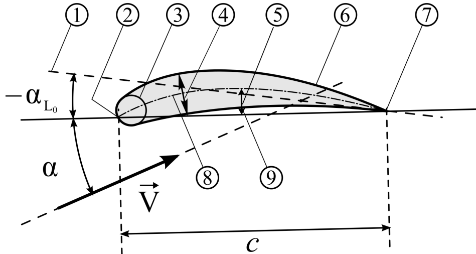
Abbildung 7.7: Geometrie der NACA Profile [37]
