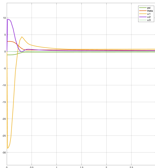
Abbildung 16.3: Simulation der Regelung mit Nachführung der K-Matrix
