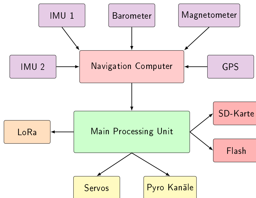
Abbildung 10.1: Systemarchitektur des Flightcomputers
