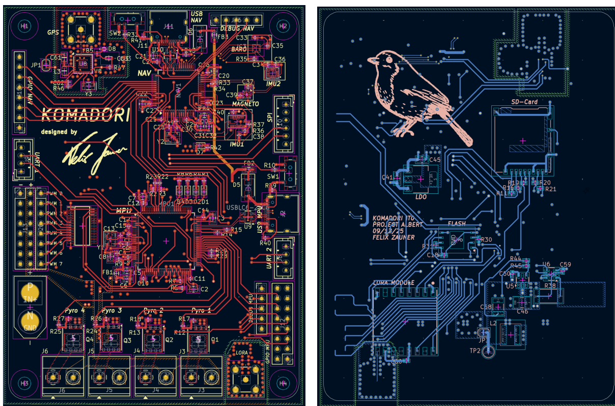
Abbildung 10.9: Layout der Leiterplatte des Flightcomputers KOMADORI (Vorder- und Rückseite)
