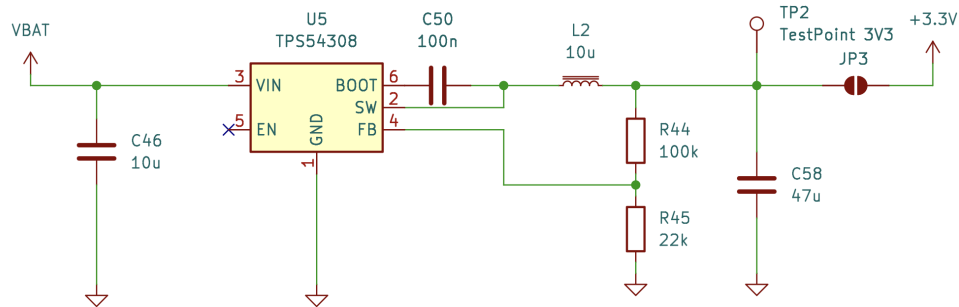
Abbildung 10.6: Schaltplan des Buck Converters basierend auf dem TPS54308
