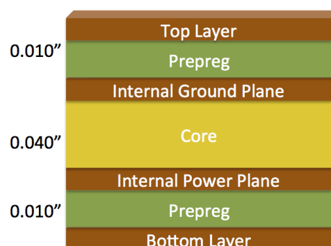
Abbildung 4.1: Beispielhafter Stackup einer vierlagigen Leiterplatte [16]
