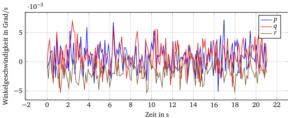
Abbildung 16.9: Rohe Gyroskopdaten der Winkelgeschwindigkeiten p , q und r
