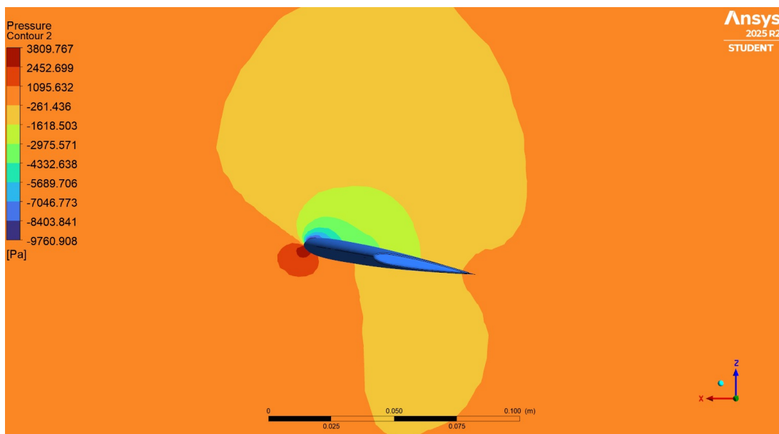
Abbildung 14.3: Druck am Raketenflügel
