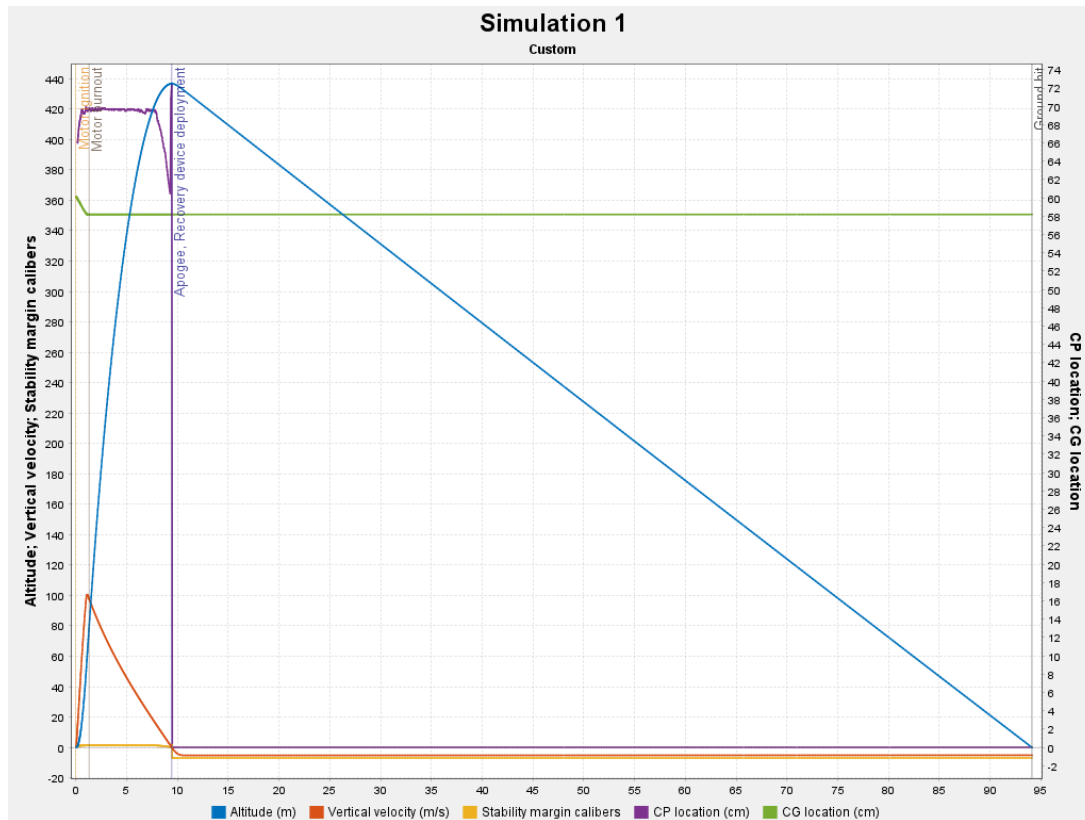
Abbildung 16.1: Plot der Simulationsergebnisse in OpenRocket
