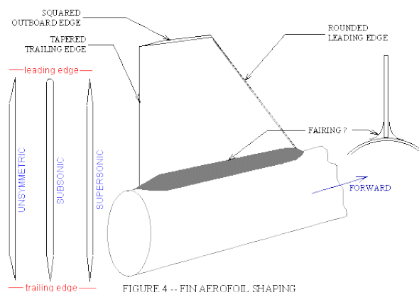
Abbildung 7.6: Flügelprofile [NakkaRocketry]
