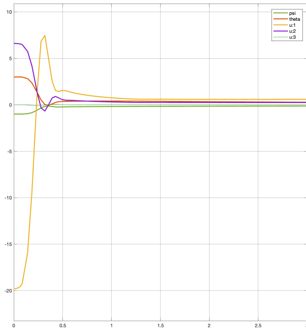
Abbildung 16.4: Simulation der Regelung ohne Nachführung der K-Matrix
