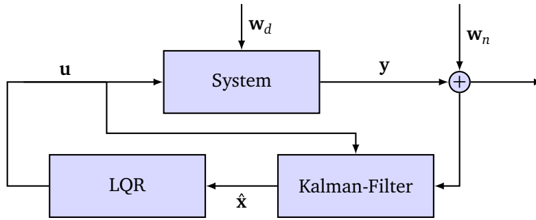
Abbildung 6.5: LQG Regler Struktur
