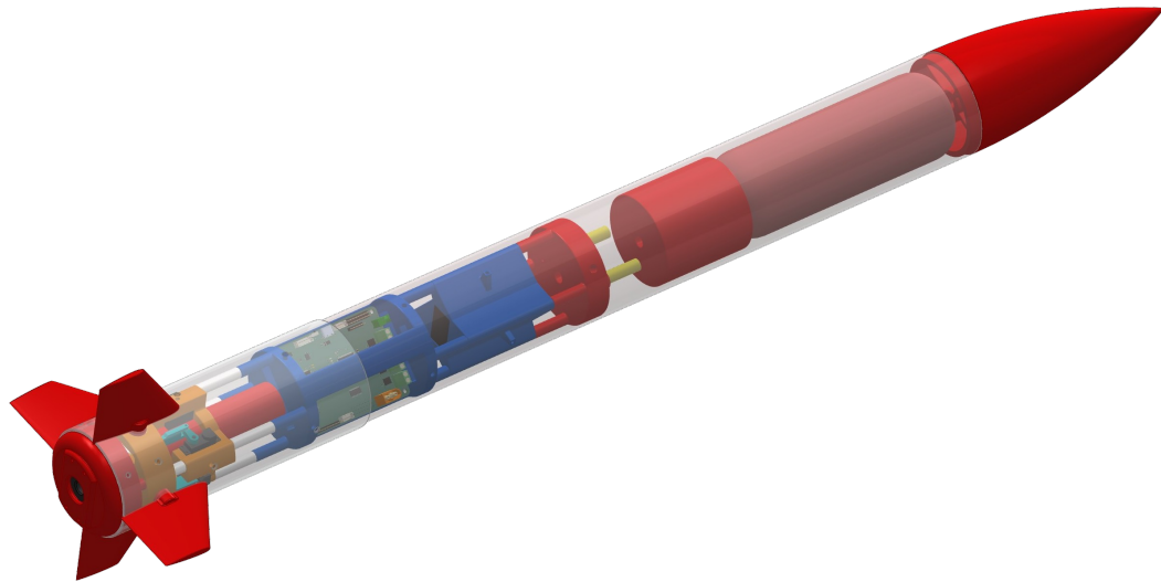
Abbildung 13.8: Zusammengesetzte CAD-Baugruppe der Rakete
