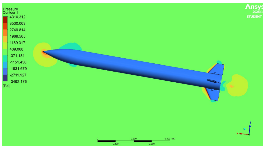
Abbildung 14.5: Druck am Raketenkörper
