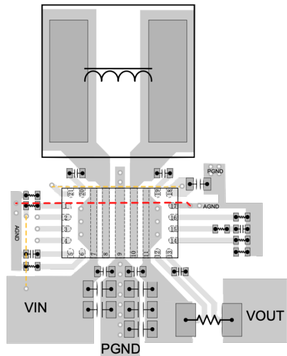
Abbildung 4.7: Beispielhaftes Layout eines Abwärtswandlers [32]
