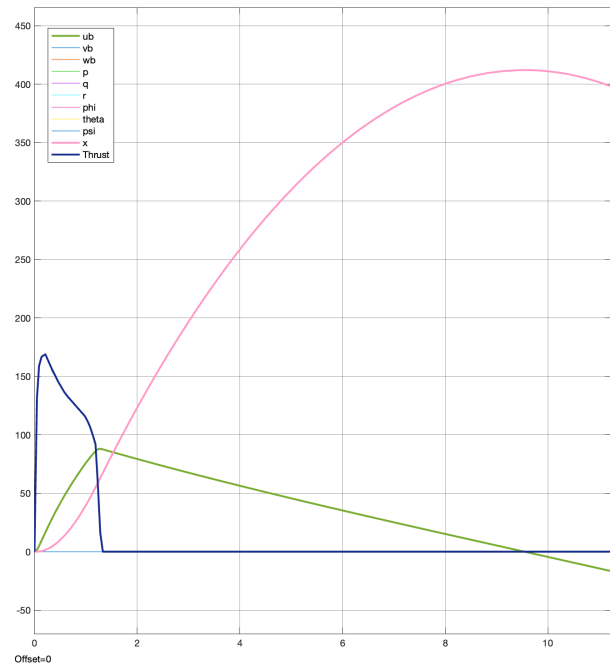
Abbildung 16.2: Ungestörter Flug der Rakete mit einem H-Motor
