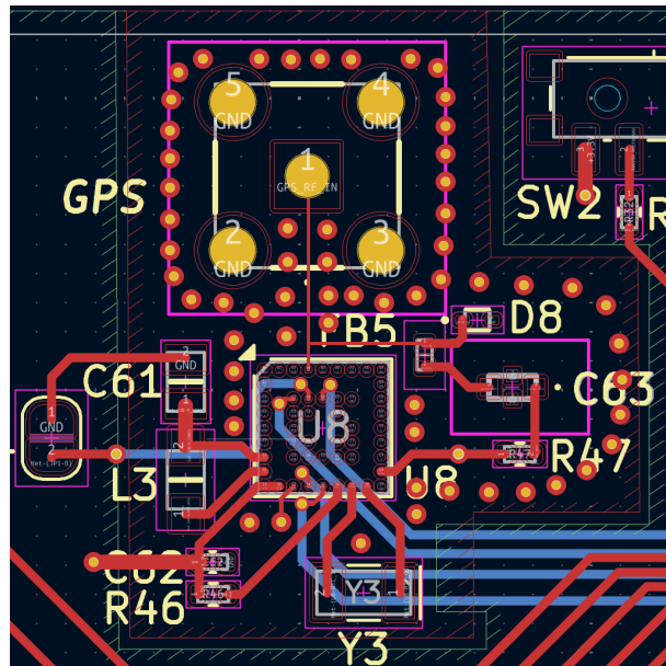
Abbildung 10.12: Layout des GPS-Moduls mit den zugehörigen Designrichtlinien
