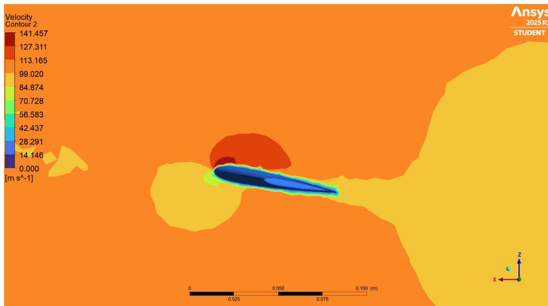
Abbildung 14.4: Geschwindigkeit am Raketenflügel
