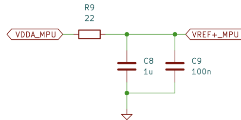
Abbildung 10.4: RC-Tiefpass zur Stabilisierung der Referenzspannung am VREF+ Pin
