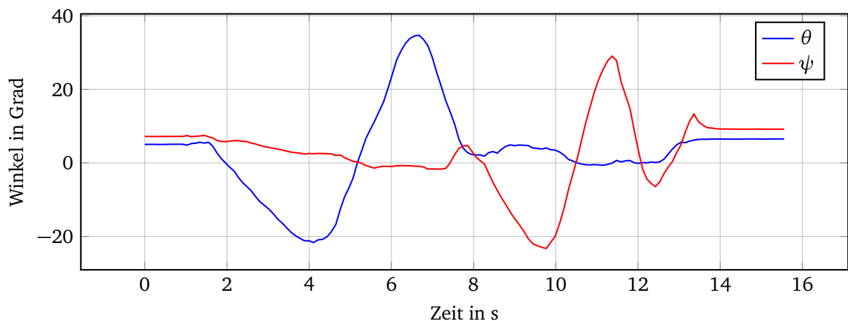
Abbildung 16.7: Verlauf der Winkel \theta und \psi
