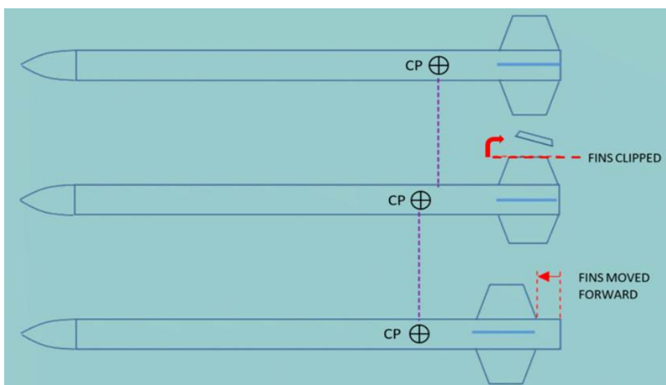
Abbildung 7.2: Verschieben des Druckpunktes durch Stutzen oder Verschieben der Flügel [26]
