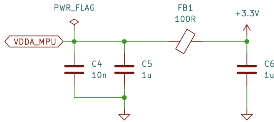
Abbildung 10.3: PI-Filter zur Entkopplung der VDDA und VREF+ Pins von der 3.3V Schiene
