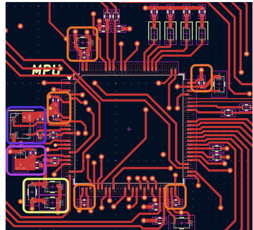
Abbildung 10.10: Layout der MPU mit den zugehörigen passiven Komponenten
