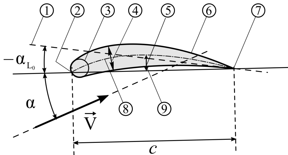
Abbildung 7.6.: Geometrie der NACA Profile [22]
