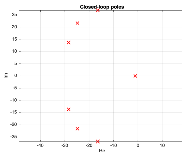
Abbildung 6.3.: Eigenwerte eines geschlossenen Regelkreises
