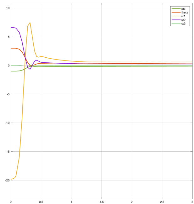
Abbildung 15.3.: Simulation der Regelung ohne Nachführung der K -Matrix
