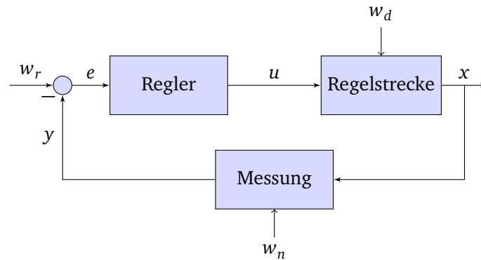
Abbildung 6.2.: Standard-Regelkreis
