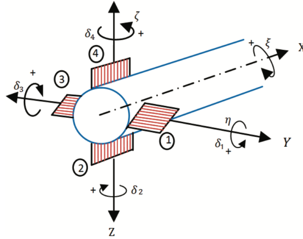
Abbildung 9.1.: Modell eines Rakete mit 6 Freiheitsgraden [8]
