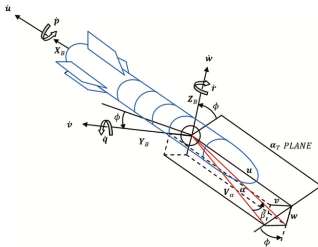
Abbildung 9.2.: Modell eines Rakete mit 6 Freiheitsgraden [8]
