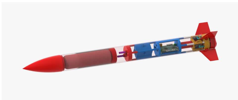
Abbildung 1: ALBERT AERO Abwehrrakete
