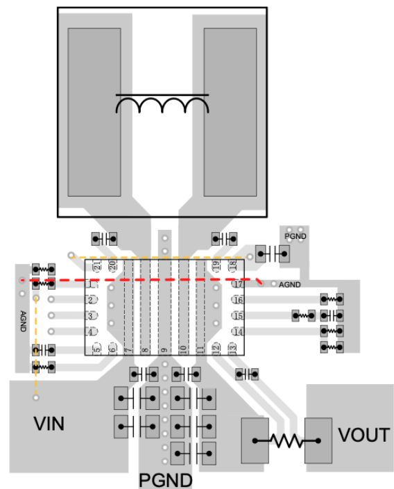
Abbildung 4.7.: Beispielhaftes Layout eines Abwärtswandlers [22]
