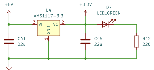
Abbildung 9.7.: Schaltplan des LDOs basierend auf dem AMS1117-3.3
