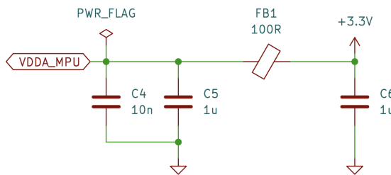
Abbildung 9.3.: PI-Filter zur Entkopplung der VDDA und VREF+ Pins von der VDD Schiene
