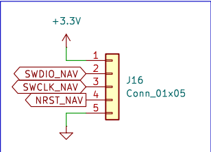
DEBUG_NAV
