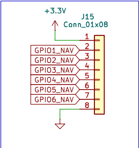
GPIO HEADER NAV
