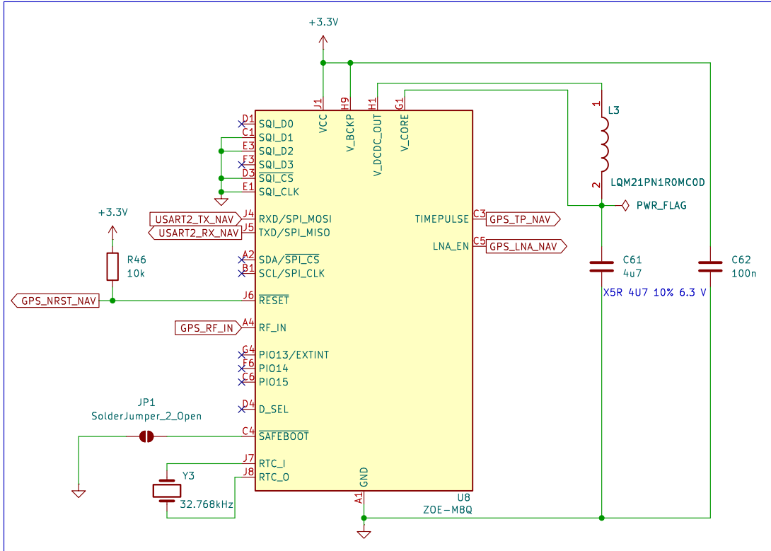
GNSS Modul
