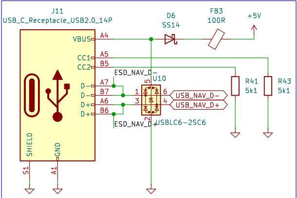
USB_NAV
