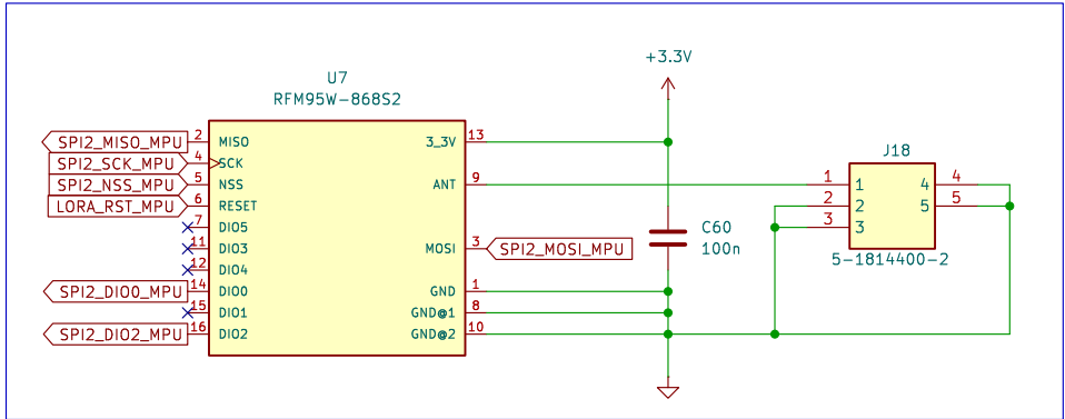
LORA Module
