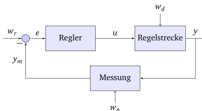
Abbildung 6.2.: Standard-Regelkreis
