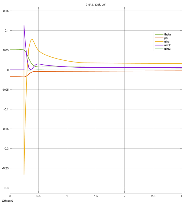
Abbildung 15.2: Ungestörter Flug der Rakete mit einem H-Motor. Im Vergleich dazu ist in Abbildung 15.3 die Simulation des gleichen Fluges dargestellt, bei dem die Regelung von Anfang an aktiv ist und die K-Matrix für die Geschwindigkeit von 50 \frac{m}{s} verwendet wird. Es ist zu erkennen, dass sich die beiden Verläufe grundsätzlich sehr ähnlich sind, die Auslenkung der Finnen jedoch merklich größer ist was zu einem Überschwinger des Winkels \theta führt. In diesem Fall ist das in Ordnung und führt zu keinerlei Problemen, da die Regelung ohnehin im Bereich unter 50 \frac{m}{s} bis ca. 1 s bleibt siehe Abbildung 15.1.
