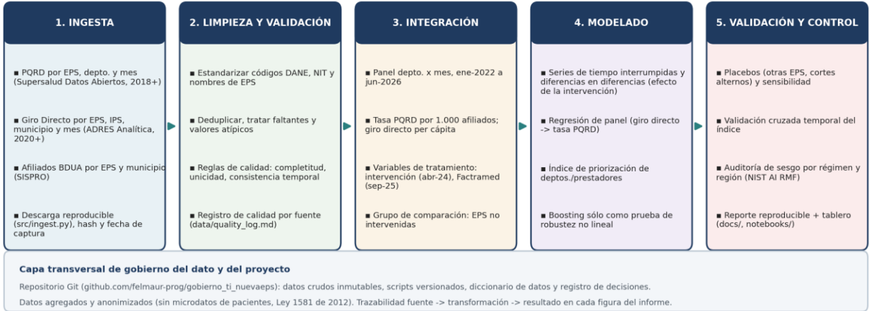
Figura 2. Pipeline de datos: ingesta -> limpieza -> integración -> modelado -> validación. Elaboración propia.
