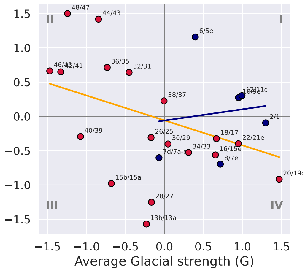
(b) SST Records
