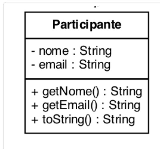
TRECHO DO DIAGRAMA DE CLASSES
