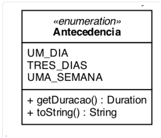
TRECHO DO DIAGRAMA DE CLASSES
