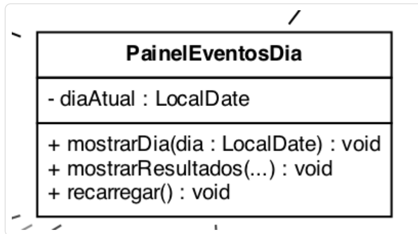
TRECHO DO DIAGRAMA DE CLASSES
