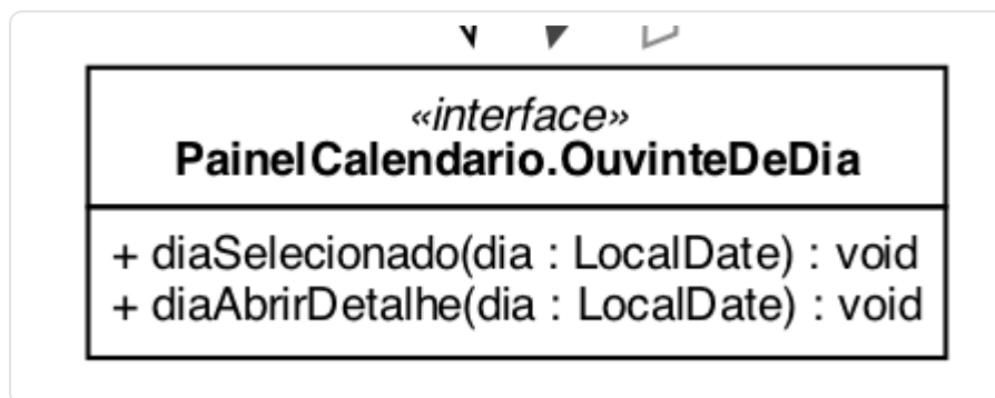
TRECHO DO DIAGRAMA DE CLASSES
