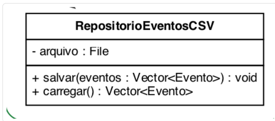
TRECHO DO DIAGRAMA DE CLASSES
