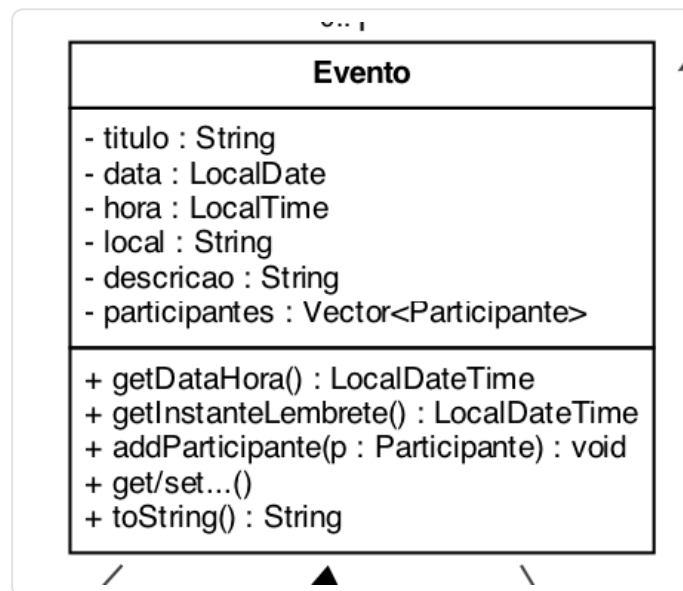
TRECHO DO DIAGRAMA DE CLASSES
