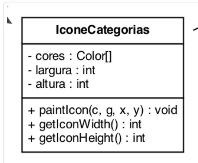
TRECHO DO DIAGRAMA DE CLASSES
