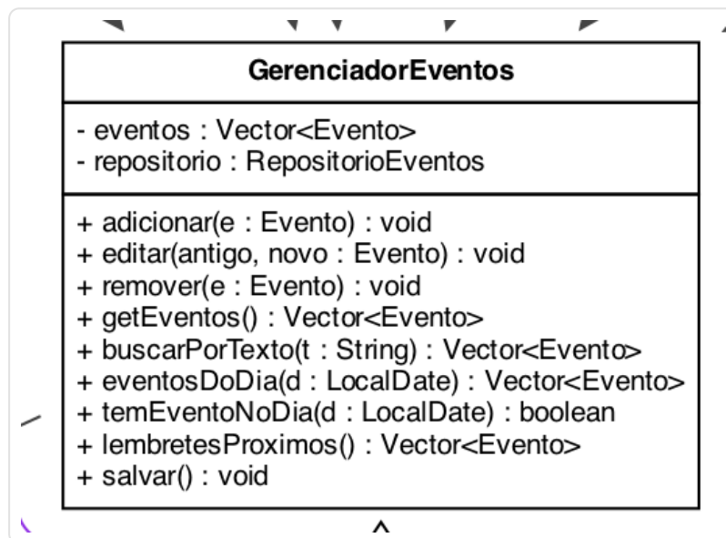
TRECHO DO DIAGRAMA DE CLASSES
