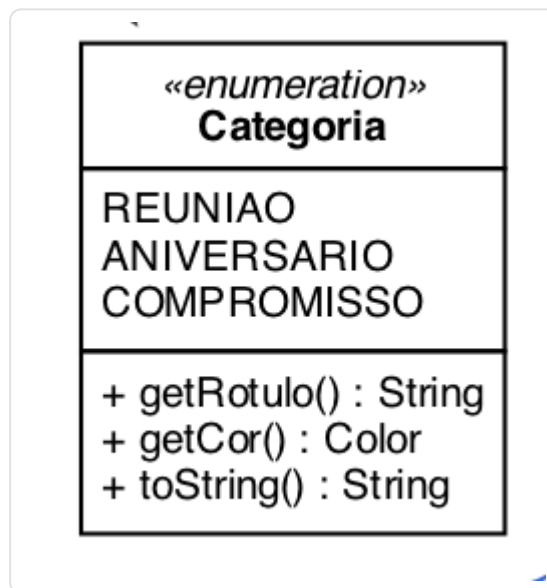
TRECHO DO DIAGRAMA DE CLASSES
