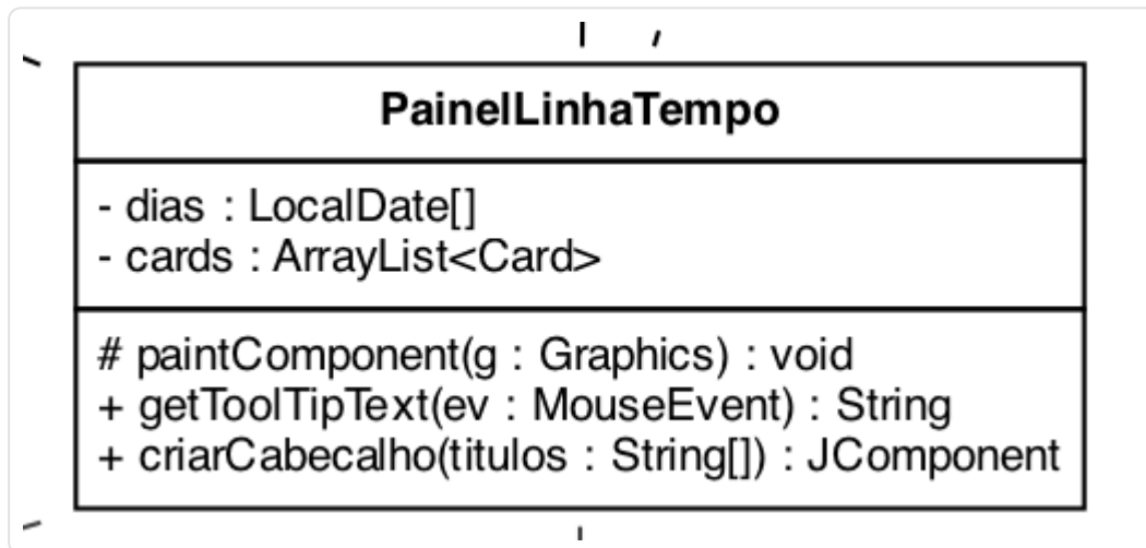
TRECHO DO DIAGRAMA DE CLASSES
