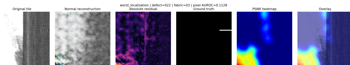
图 9 AITEX 切边缺陷 0104_022_03 的较差定位案例，单图 Pixel AUROC 仅为 0.1128。热图主要响应正常纹理而非真实缺陷，反映 64 \times 64 输入分辨率、材质域偏移及单尺度窗口共同造成的定位失败。
