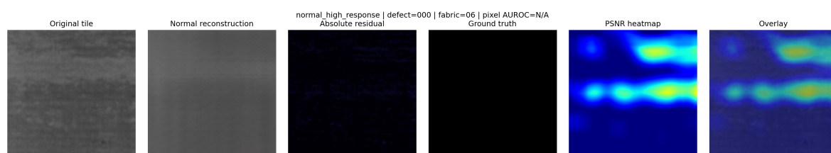
图 12 AITEX 域内训练后的正常高响应案例 0017_000_06。该图不存在真实缺陷，但周期纹理和亮度带仍产生连续高响应；逐图 min-max 归一化进一步放大了这种相对误差。
